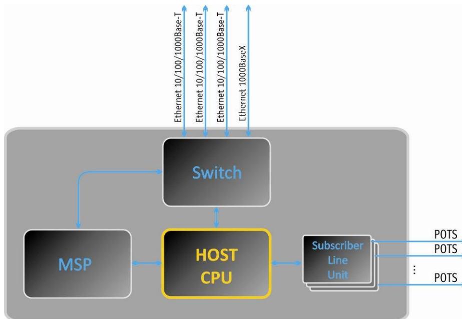
Рисунок 3 – Функциональная схема TAU-72.IP
