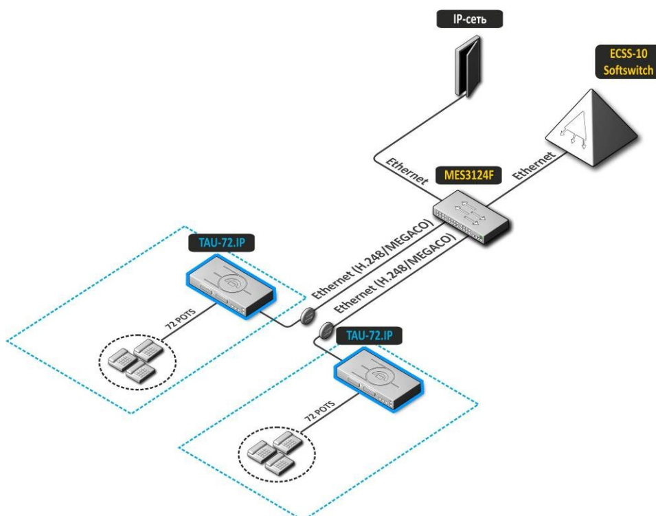
Рисунок 2 – Распределенная миниАТС TAU-72.IP
