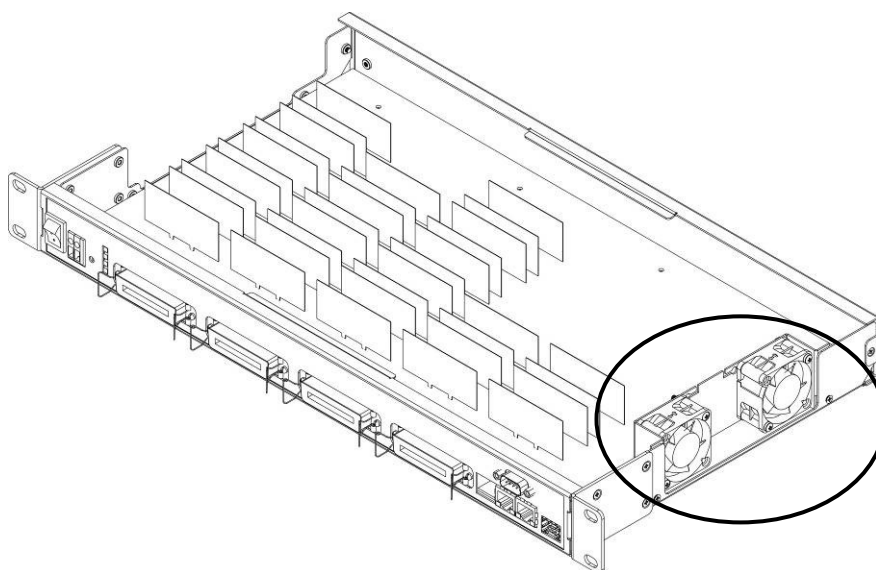
Рисунок 6 – Расположение вентиляторов
