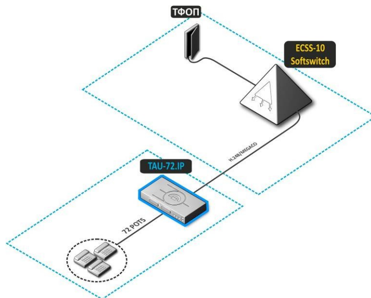
Рисунок 1 – Абонентский вынос TAU-72.IP
