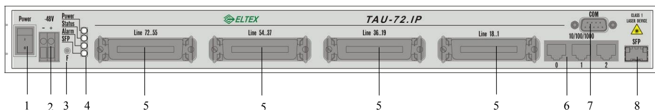
Рисунок 4 – Внешний вид передней панели TAU-72.IP.
