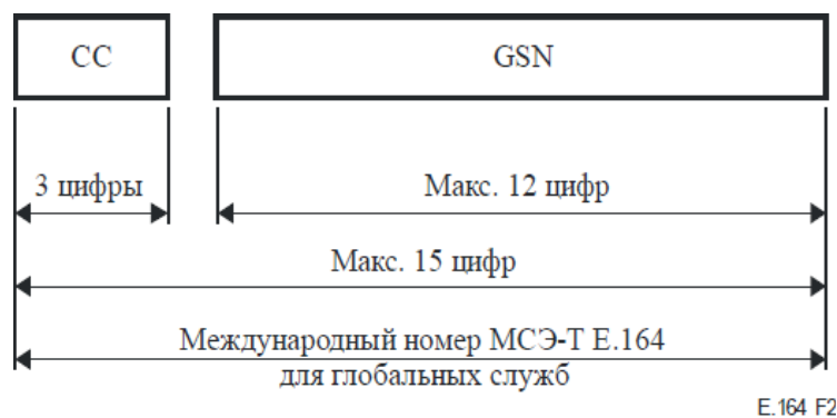
Рисунок 1.10 – Структура международного номера E.164 для глобальных услуг
