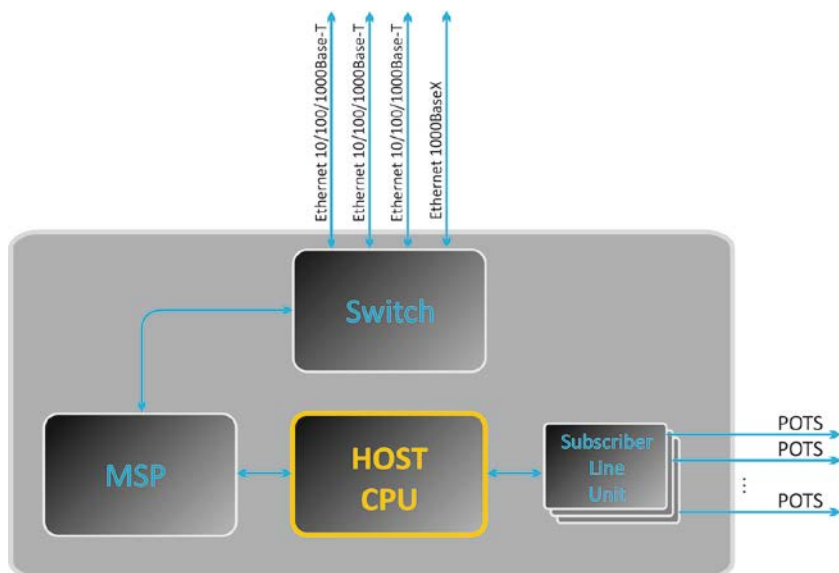
Рисунок 3а – Функциональная схема TAU-72.IP
