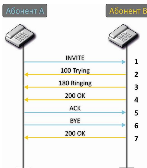
Рисунок 11 – Алгоритм вызова по протоколу SIP
