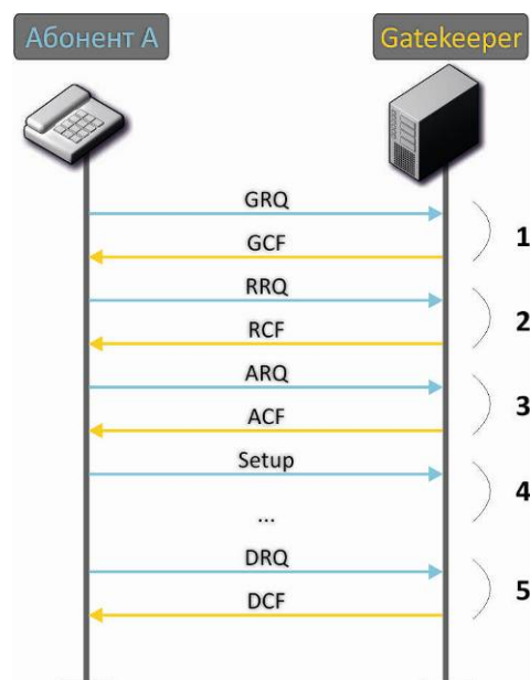
Рисунок 15 – Алгоритм вызова через гейткипер
