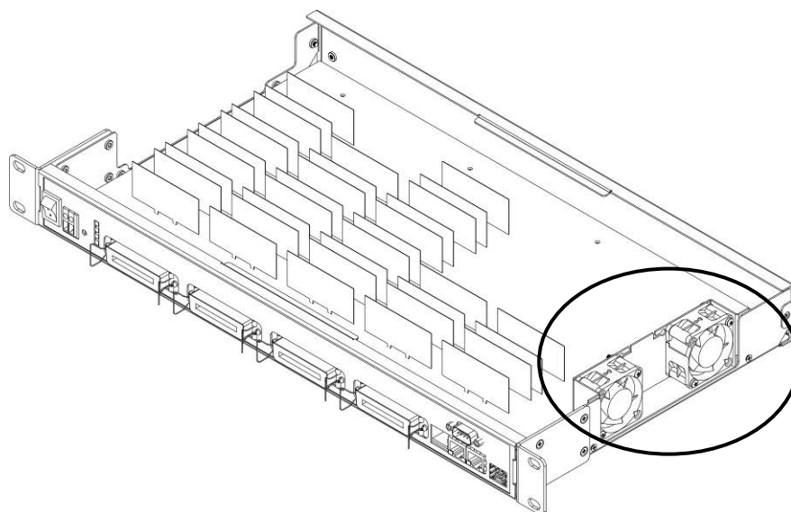
Рисунок 6 – Расположение вентиляторов
