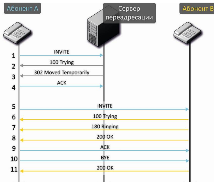
Рисунок 13 – Алгоритм вызова с участием сервера переадресации
