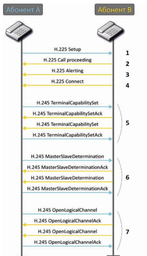
Рисунок 14 – Алгоритм вызова по протоколу H.323
