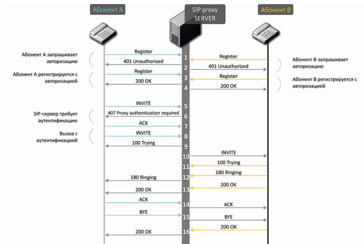
Рисунок 12 – Алгоритм вызова с участием SIP проху-сервера
