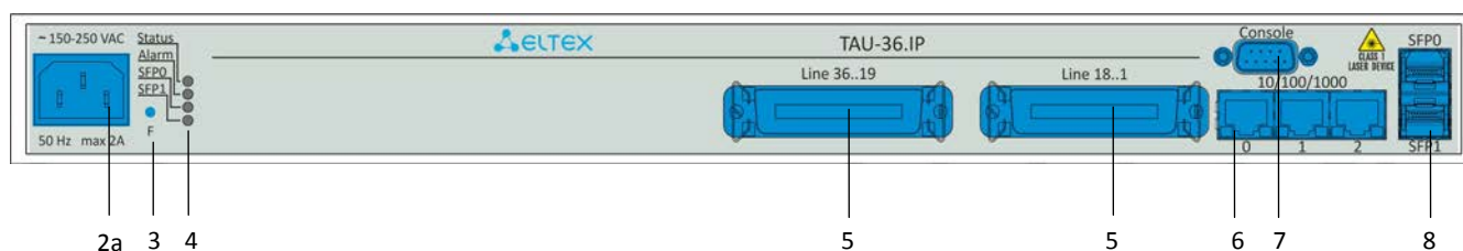
Рисунок 4е – Внешний вид передней панели TAU-36.IP с питанием от сети переменного тока
