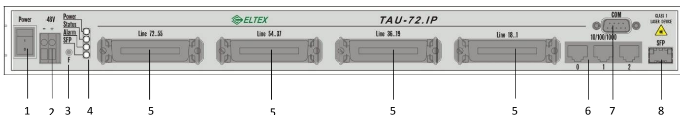
Рисунок 4а – Внешний вид передней панели TAU-72.IP v2.0
