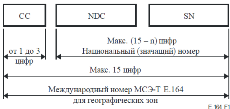
Рисунок 1.9 – Структура международного номера E.164 для географических зон
