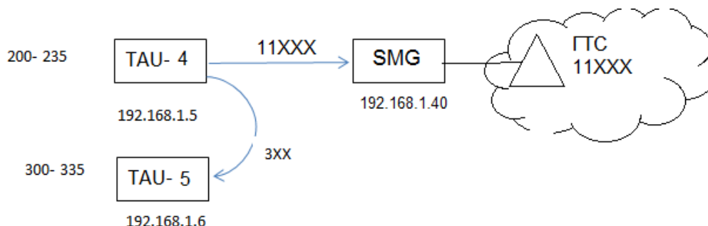
Рисунок 2.9 – Фрагмент сети 2
