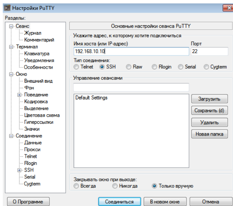
Рисунок 2 – Запуск SSH-клиента
