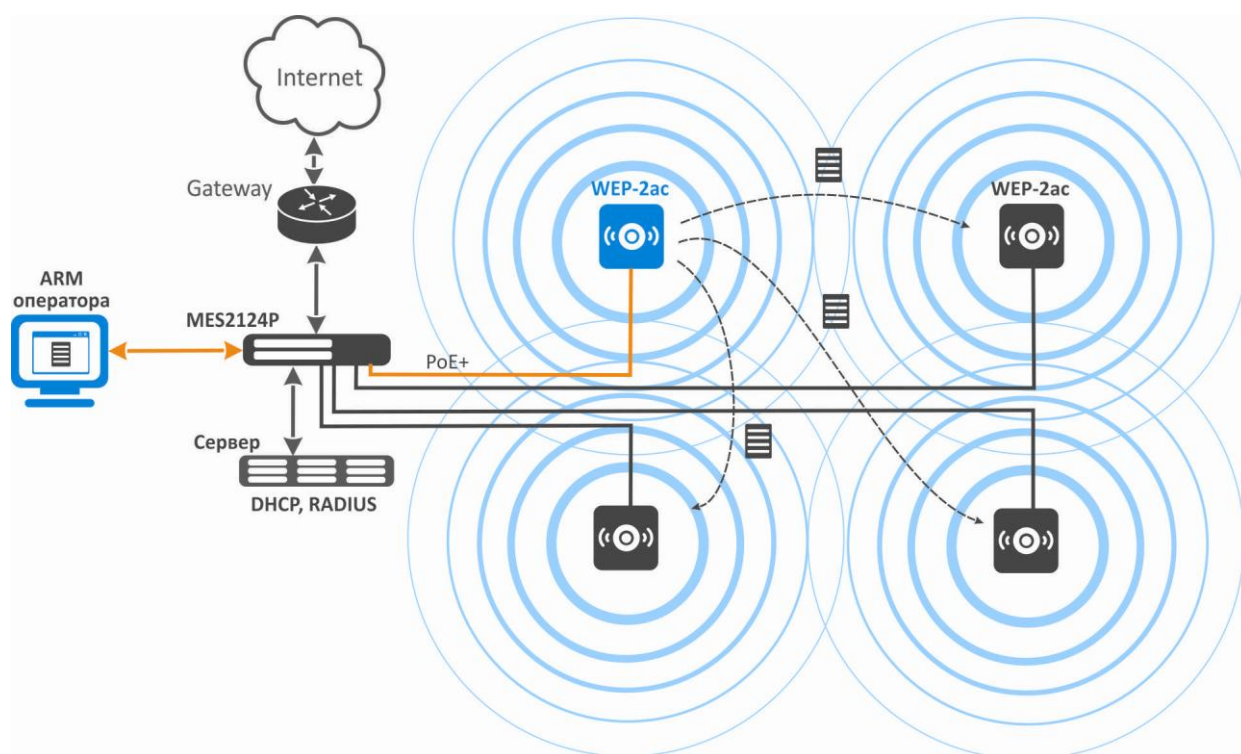
Рисунок 1 – Функциональная схема использования WEP-2ac
