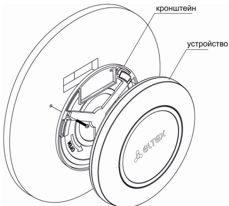
Рисунок 8 – Установка устройства (вид спереди)
