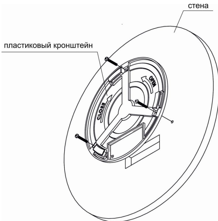
Рисунок 7 – Крепление кронштейна на стене
