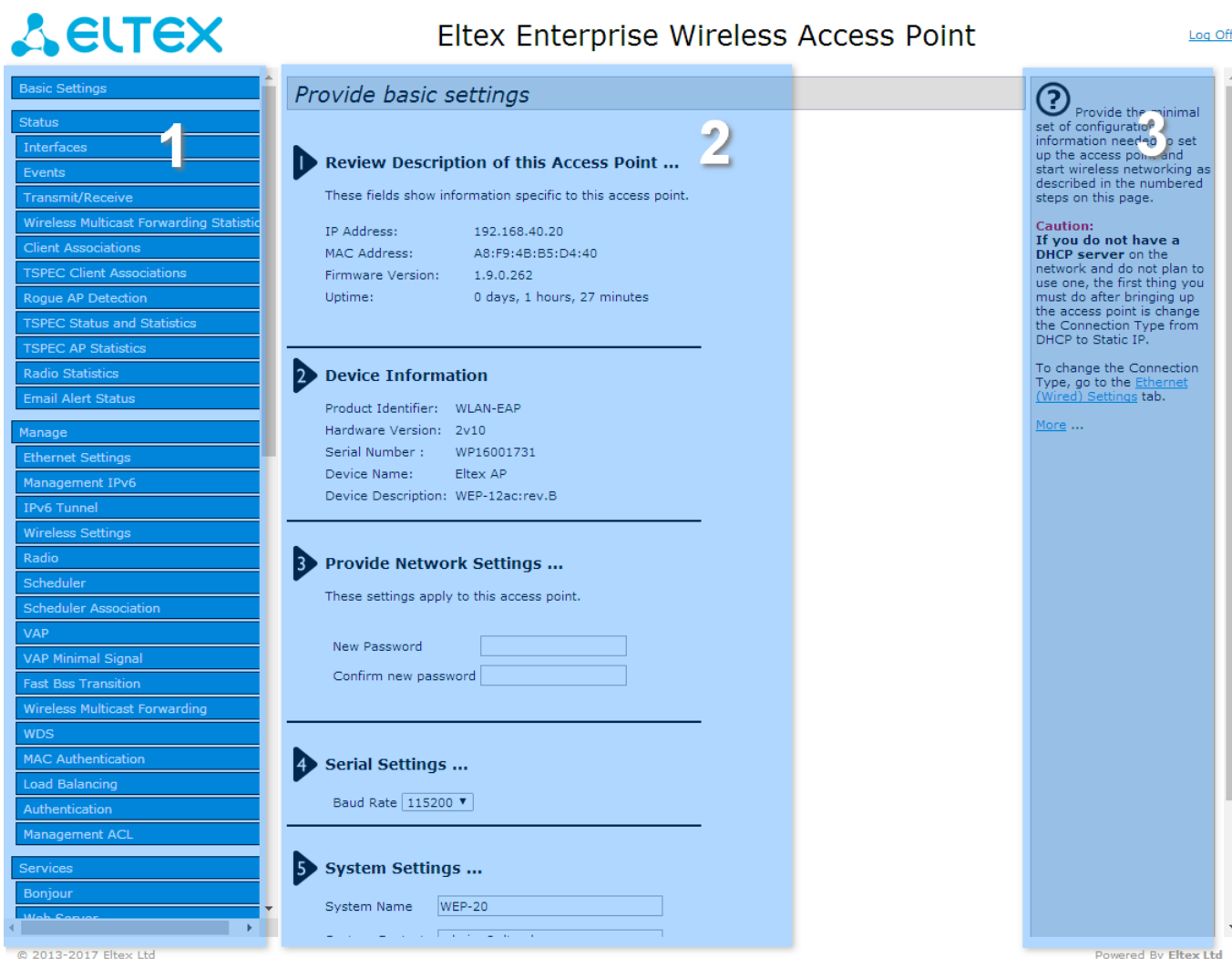
Рисунок 1 – Элементы навигации Web-конфигуратора
