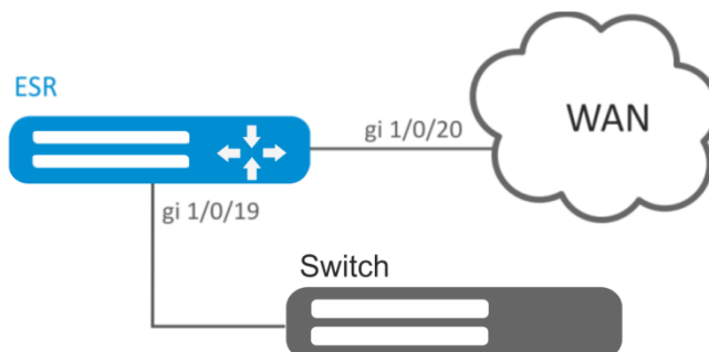
Рисунок 7.27 – Схема сети
