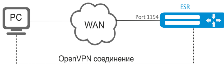
Рисунок 7.24 – Схема сети
