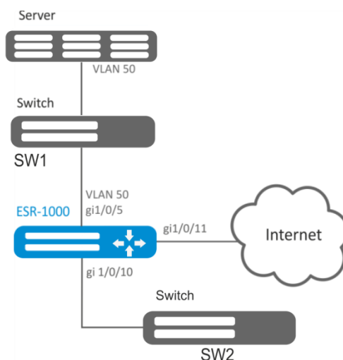
Рисунок 7.28 – Схема сети
