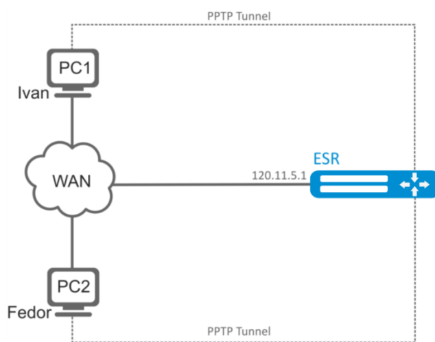
Рисунок 7.22 – Схема сети
