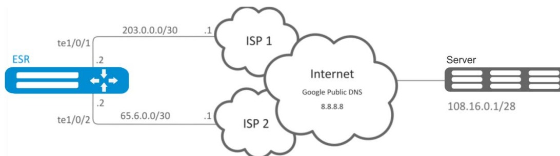
Рисунок 7.36 – Схема сети
