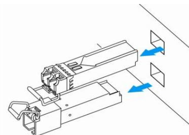
Рисунок 3.8 – Извлечение SFP-трансиверов
