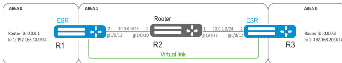
Рисунок 7.15– Схема сети
