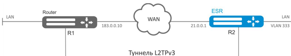
Рисунок 7.20 – Схема сети
