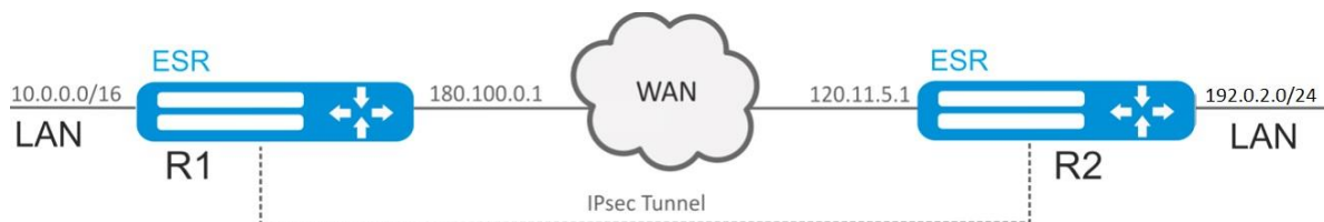
Рисунок 7.21– Схема сети
