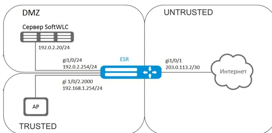
Рисунок 7.388 – Схема сети
