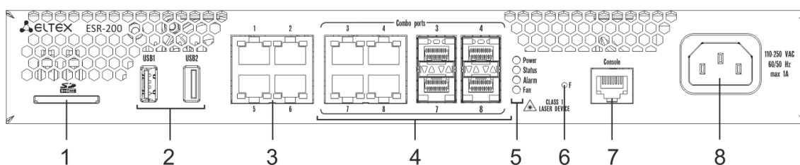
Рисунок 2.7 – Передняя панель ESR-200
