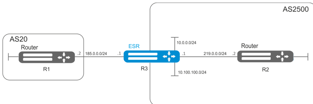
Рисунок 7.17 – Схема сети
