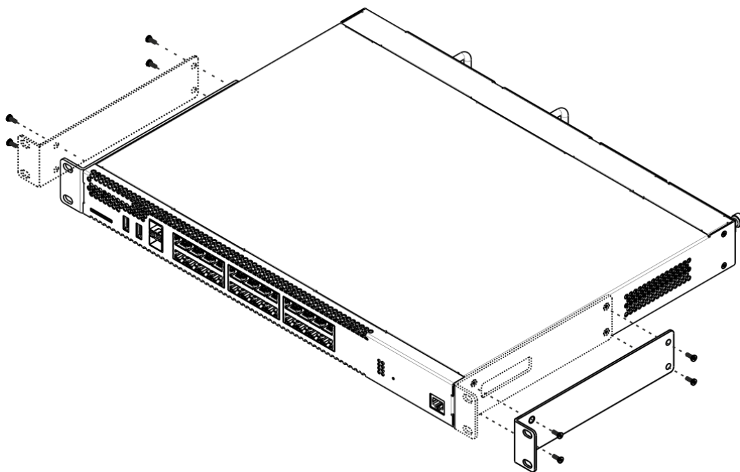
Рисунок 3.1 – Крепление кронштейнов
