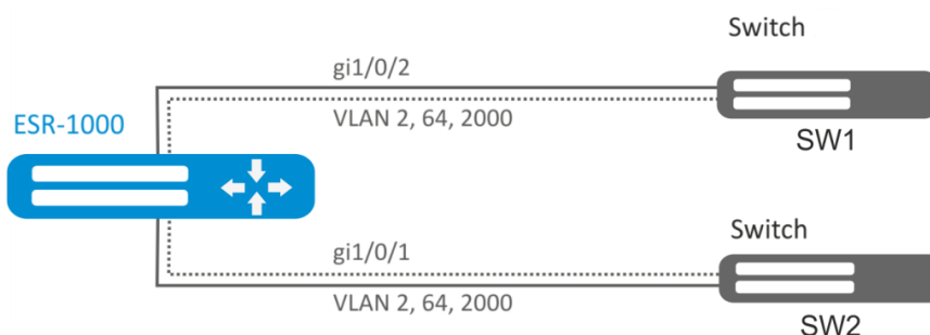
Рисунок 7.2 – Схема сети
