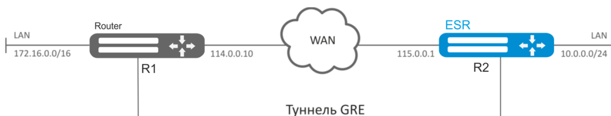
Рисунок 7.19 – Схема сети
