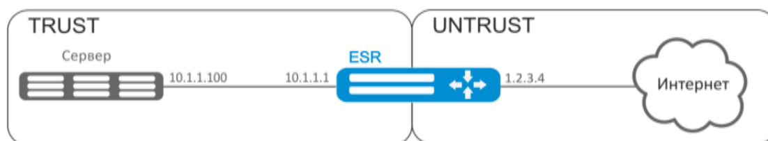
Рисунок 7.4– Схема сети
