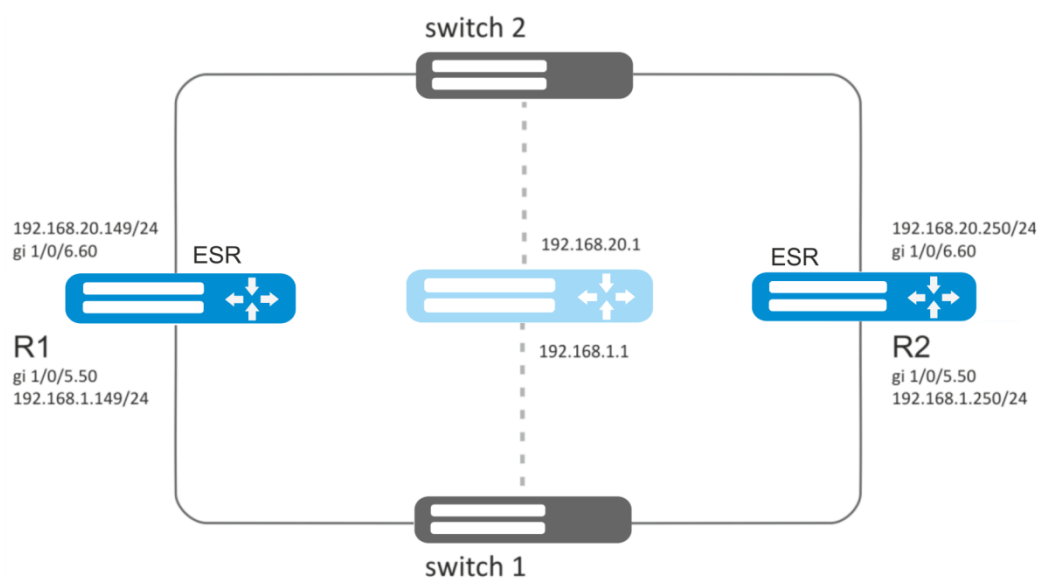
Рисунок 7.33 – Схема сети
