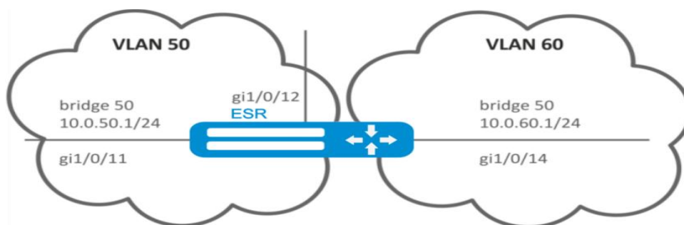
Рисунок 7.11 – Схема сети
