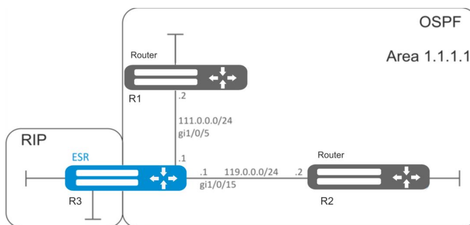
Рисунок 7.13 – Схема сети
