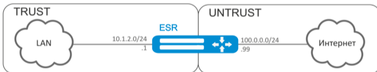
Рисунок 7.5 – Схема сети
