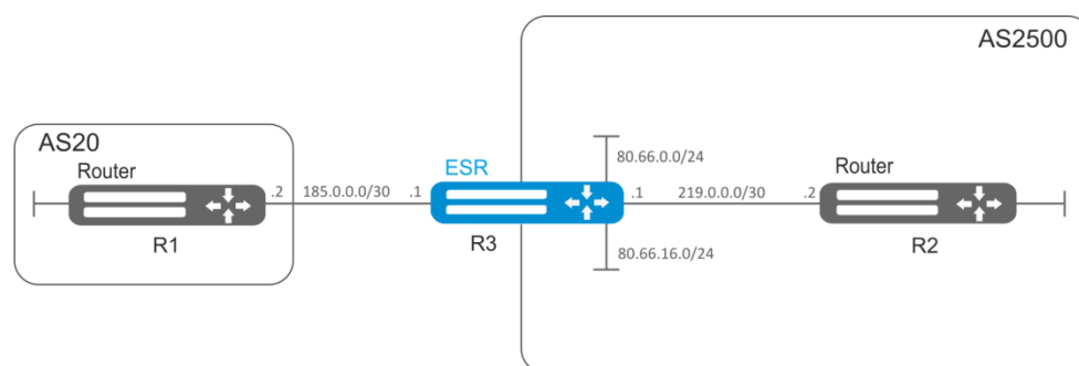
Рисунок 7.16– Схема сети
