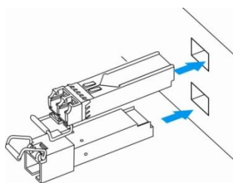
Рисунок 3.5 – Установка SFP-трансиверов
