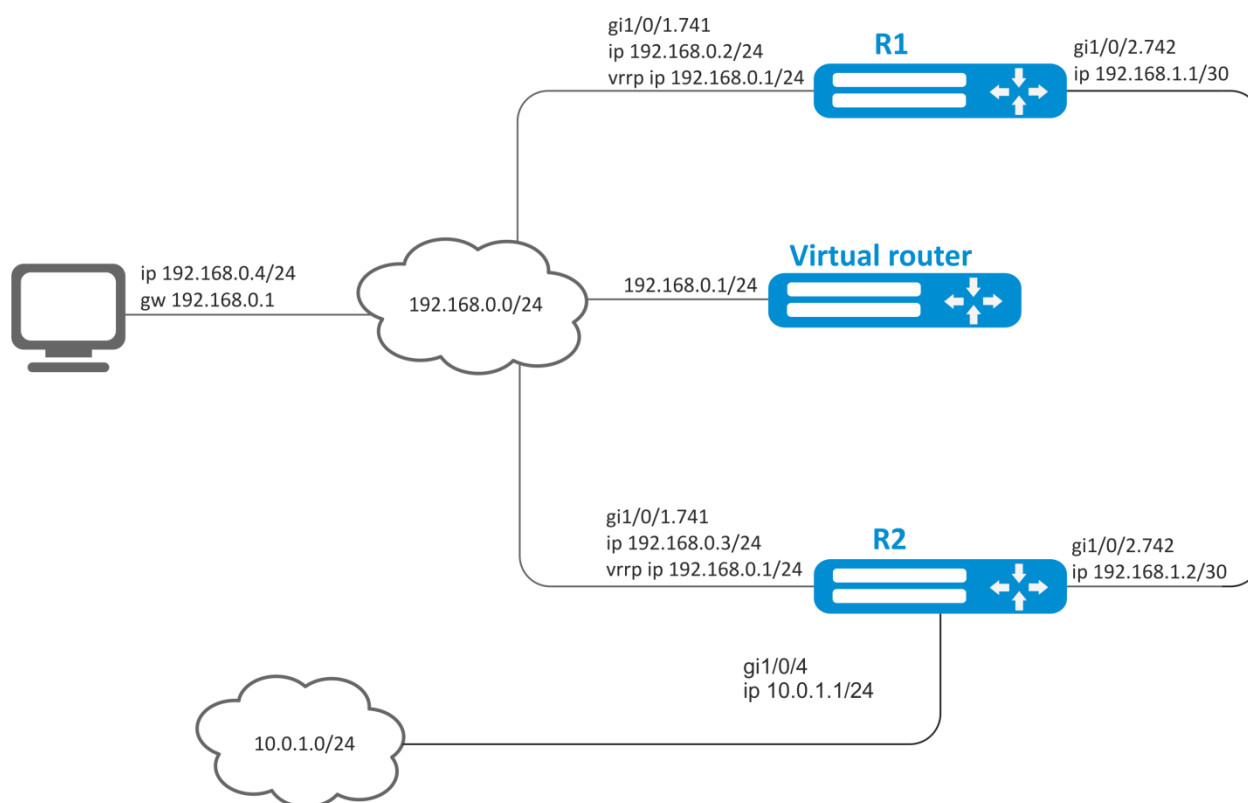
Рисунок 7.34 – Схема сети
