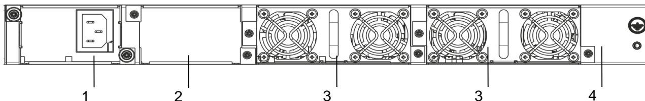
Рисунок 2.3 – Задняя панель ESR-1000, ESR-1200
