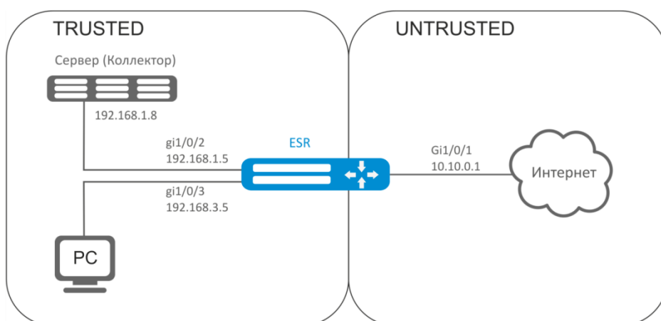
Рисунок 7.30 – Схема сети
