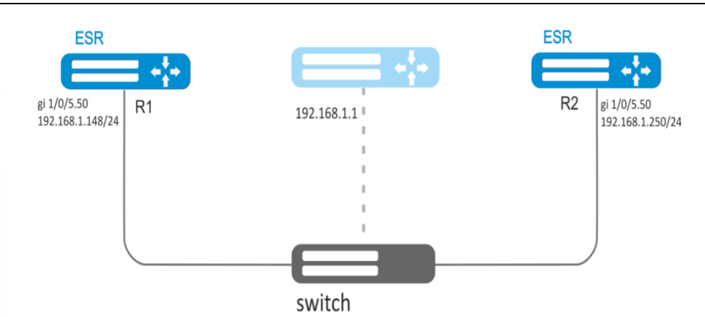
Рисунок 7.32 – Схема сети
