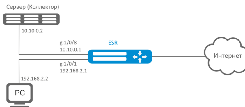
Рисунок 7.29 – Схема сети
