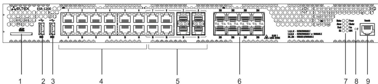
Рисунок 2.1 – Передняя панель ESR-1200
