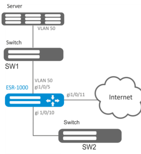
Рисунок 7.28 – Схема сети
