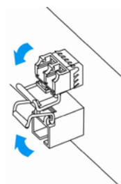
Рисунок 15 – Открытие защелки SFP-трансиверов
