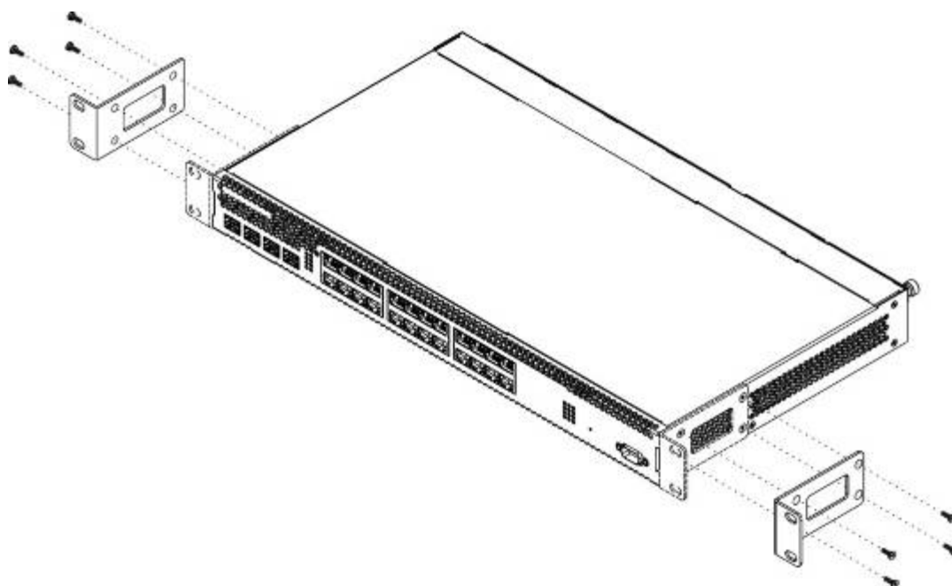
Рисунок 9— Крепление кронштейнов
