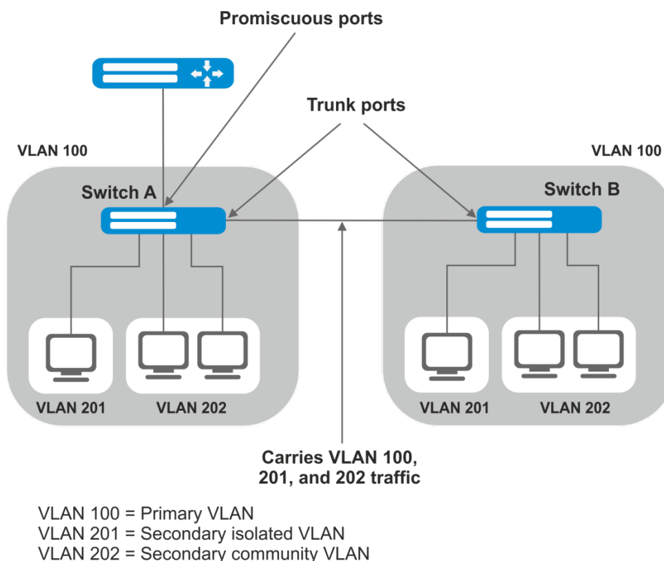
Рисунок 23 – Пример работы технологии Private VLAN
