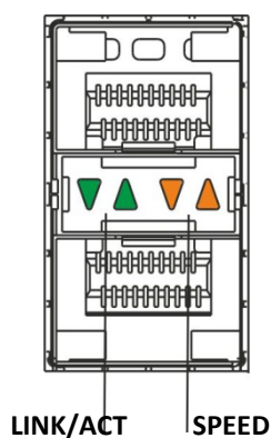
Рисунок 13– Внешний вид разъема с SFP-трансиверами
