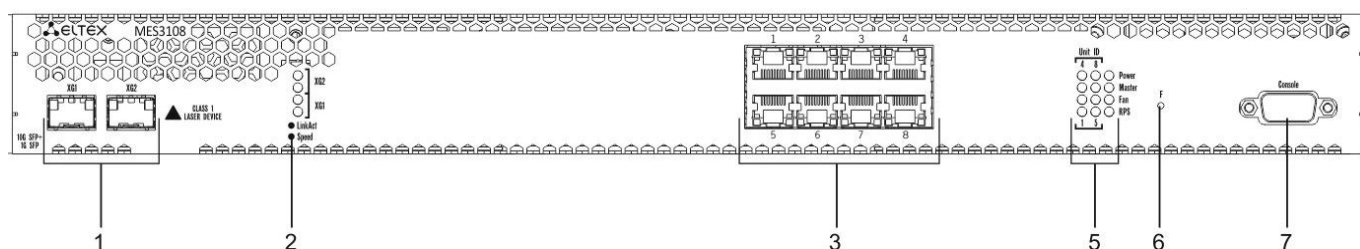
Рисунок 1 – MES3108, передняя панель
