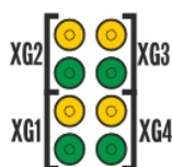
Рисунок 14 – Внешний вид индикаторов интерфейсов XG
