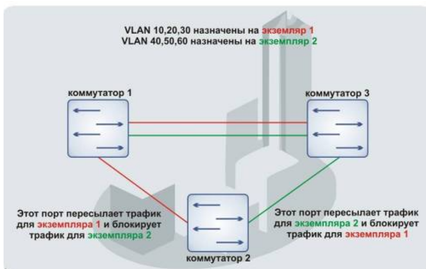
Рисунок 25 - Настройка протокола множества связующих деревьев
