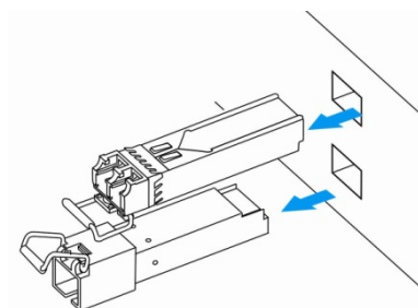
Рисунок 22 – Извлечение SFP-трансиверов
