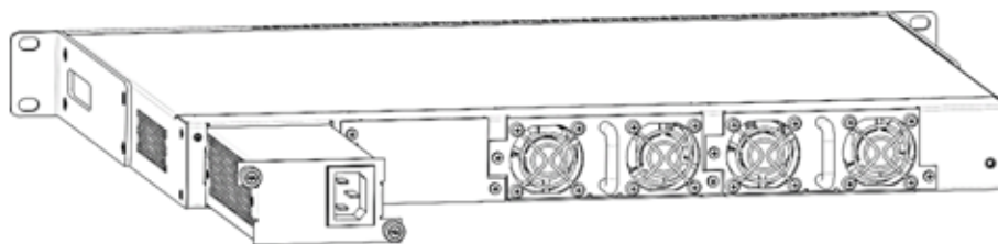
Рисунок 60 – Установка модулей питания
