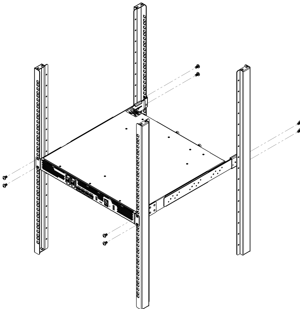
Рисунок 59 – Установка ESR-3300 в стойку
