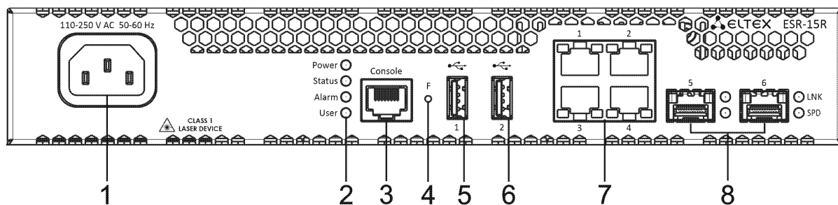
Рисунок 40 – Передняя панель ESR-15R
