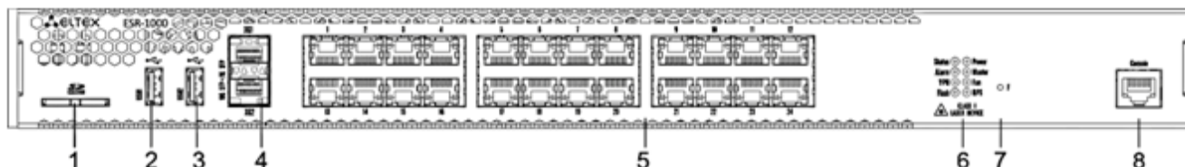
Рисунок 18 – Передняя панель ESR-1000
