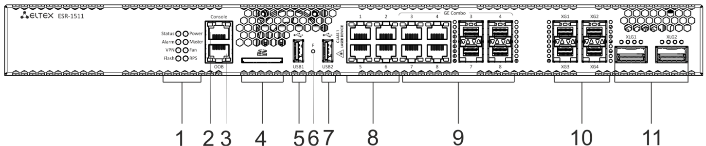
Рисунок 13 – Передняя панель ESR-1511
