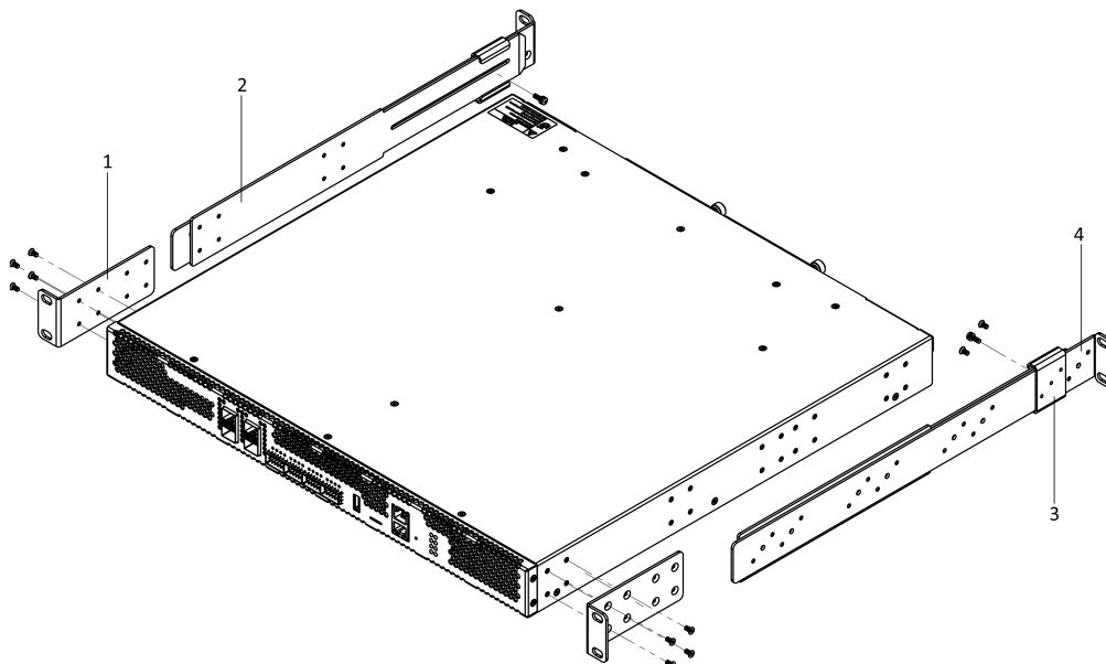
Рисунок 58 – Крепление кронштейнов к ESR-3300
