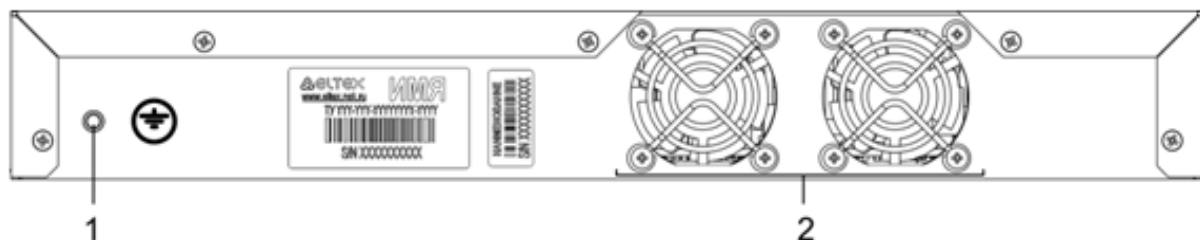
Рисунок 24 – Задняя панель ESR-200, ESR-100
