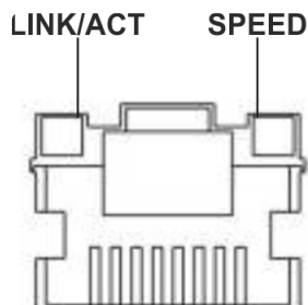
Рисунок 44 – Расположение индикаторов разъема RJ-45
