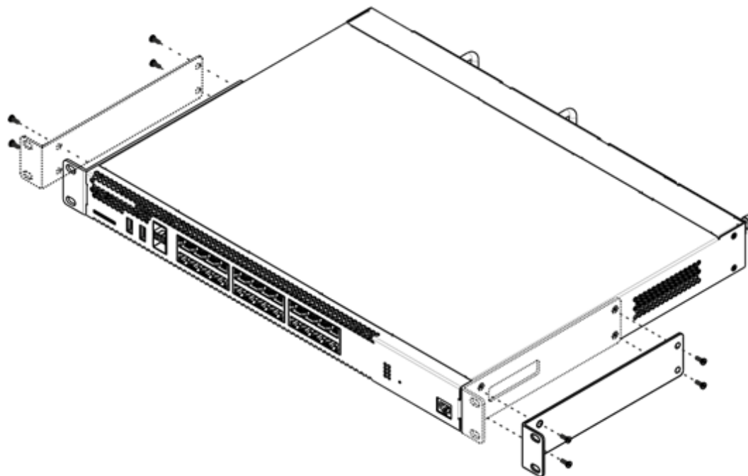
Рисунок 56 – Крепление кронштейнов к устройству
