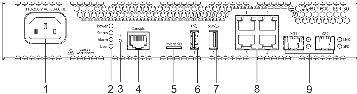
Рисунок 35 – Передняя панель ESR-30
