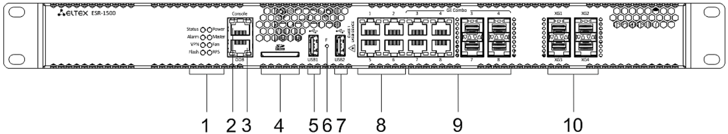
Рисунок 14 – Передняя панель ESR-1500
