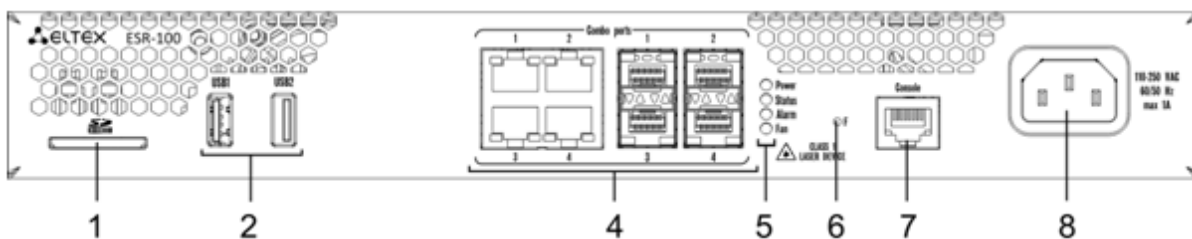
Рисунок 23 – Передняя панель ESR-100
