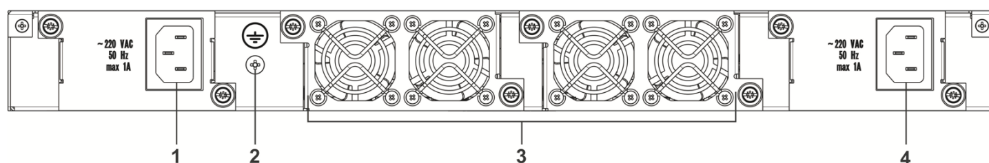
Рисунок 15 – Задняя панель ESR-1511, ESR-1500
