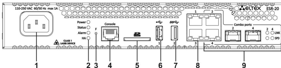
Рисунок 36 – Передняя панель ESR-20
