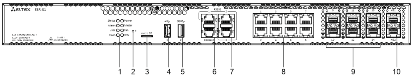
Рисунок 27 – Передняя панель ESR-31
