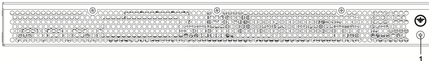
Рисунок 32 – Задняя панель ESR-21
