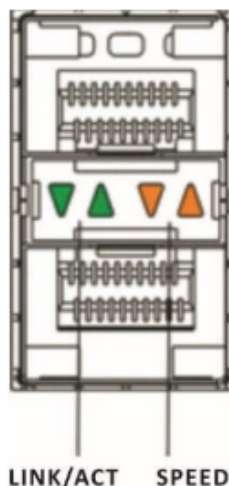
Рисунок 45 – Расположение индикаторов SFP/SFP+/SFP28-интерфейсов
