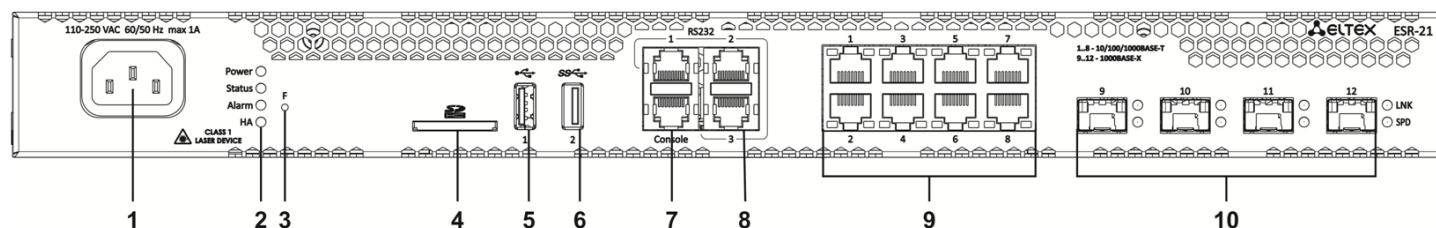
Рисунок 31 – Передняя панель ESR-21
