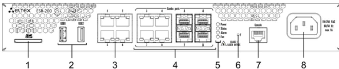
Рисунок 22 – Передняя панель ESR-200
