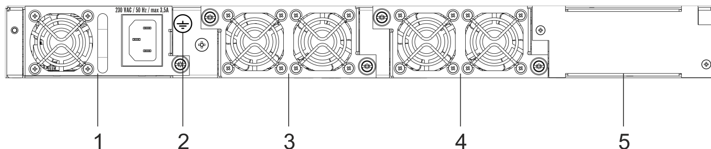
Рисунок 10 – Задняя панель ESR-3200
