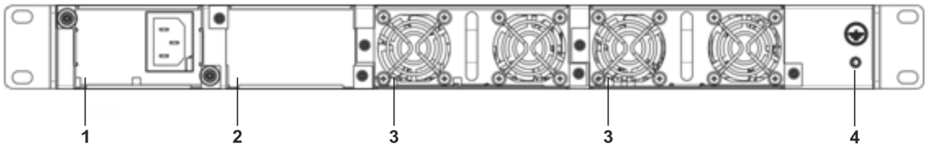
Рисунок 19 – Задняя панель ESR-1000
