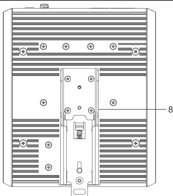
Рисунок 58 – Задняя панель MES3500I-8P8F
