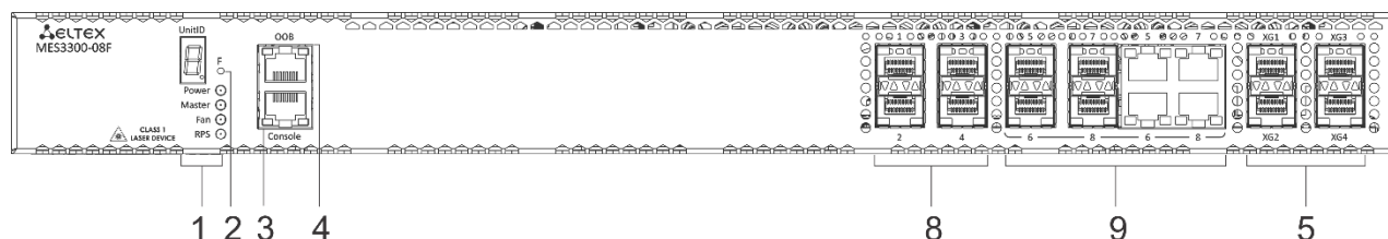
Рисунок 17 – Передняя панель MES3300-08F
