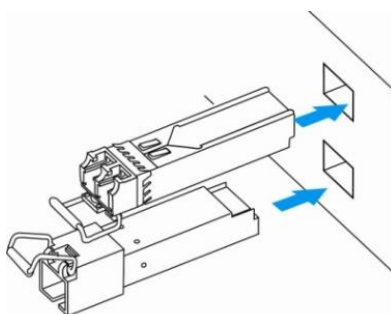
Рисунок 110 – Установка SFP-трансиверов
