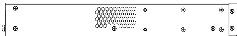
Рисунок 70 – Левая боковая панель MES2300-24F
