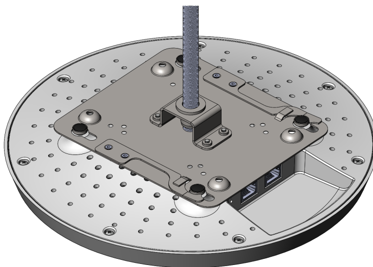
Рисунок 19 — Фиксация устройства на монтажной пластине
