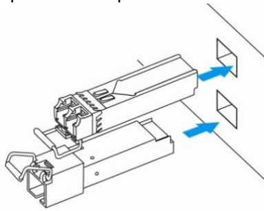
Рисунок 60 – Установка SFP-трансиверов
