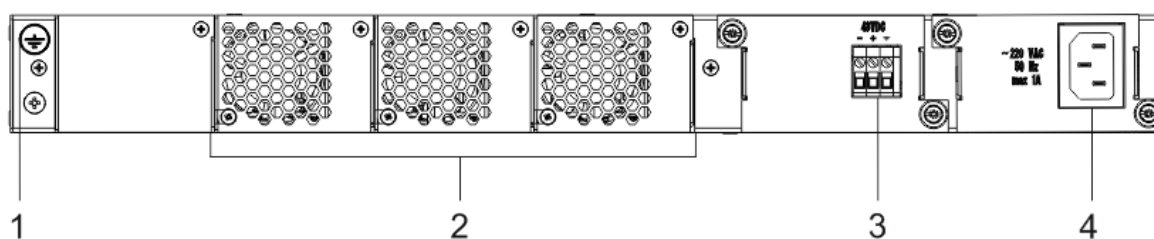
Рисунок 27 — Задняя панель MES3316F
