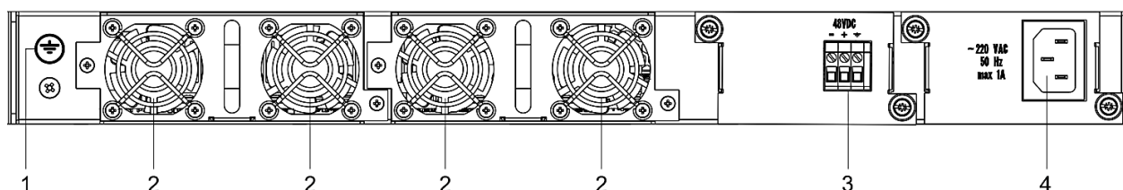
Рисунок 25 — Задняя панель MES5324
