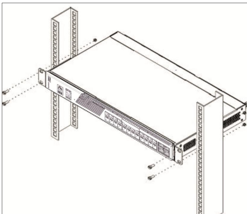
Рисунок 21– Установка устройства в стойку
