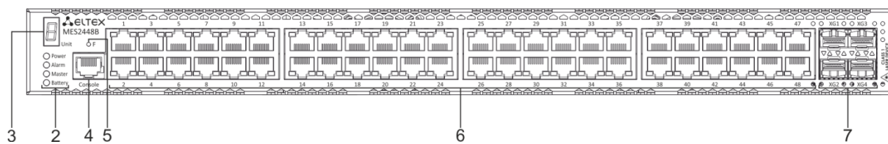
Рисунок 22 – Передняя панель MES2448B
