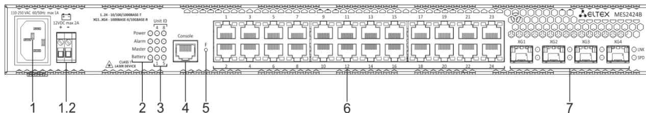
Рисунок 19 – Передняя панель MES2424B
