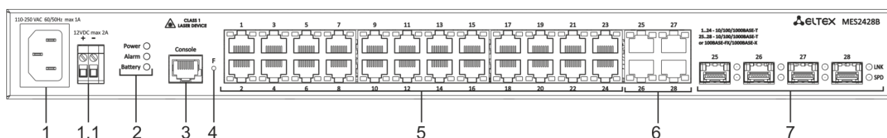
Рисунок 14 – Передняя панель MES2428B
