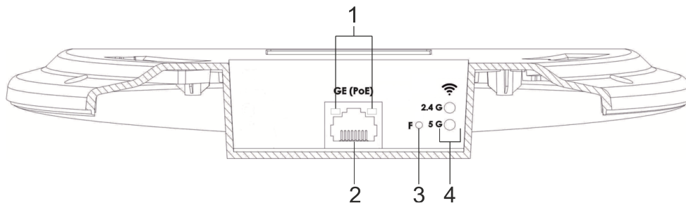
Рисунок 2 – Внешний вид основной панели WEP-3L
