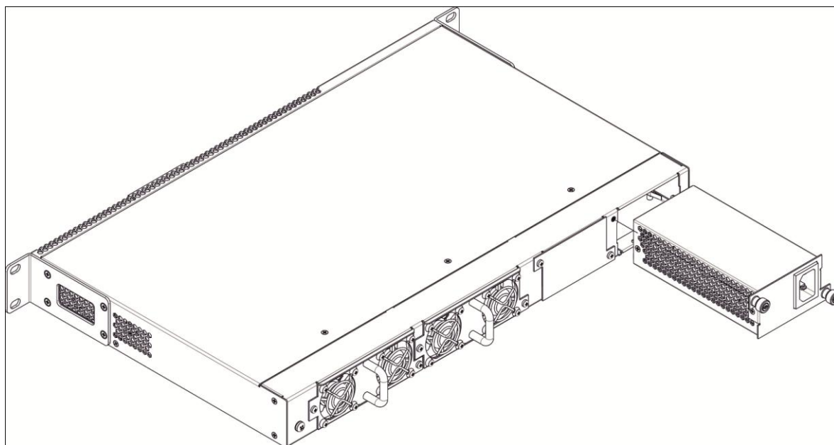
Рисунок 23 – Установка модулей питания.
