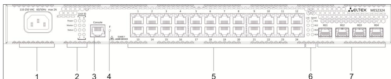
Рисунок 3 – MES2324, передняя панель
