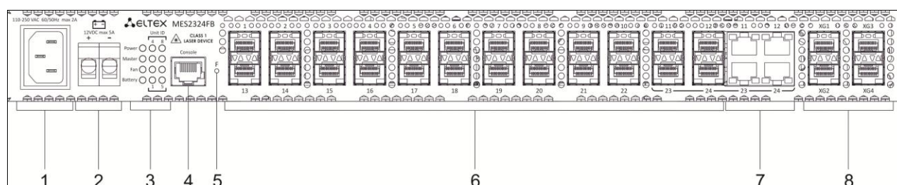
Рисунок 5 – MES2324FB, передняя панель
