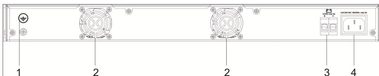
Рисунок 13 – MES2348B, задняя панель
