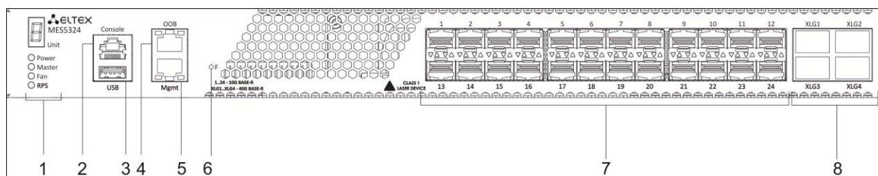
Рисунок 1– MES5324, передняя панель
