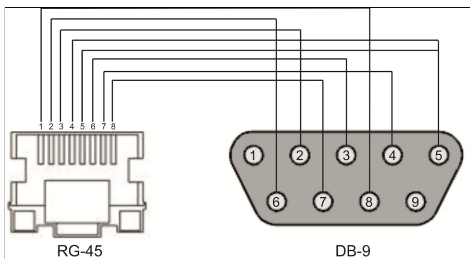
Рисунок 26 - Подключение консольного кабеля
