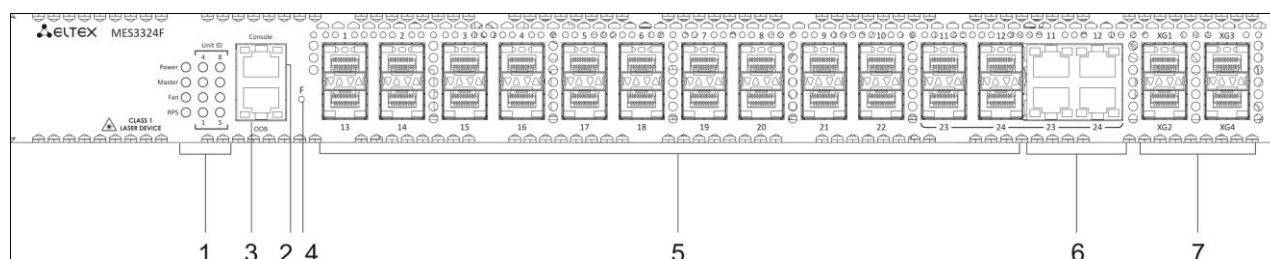
Рисунок 2 – MES3324F, передняя панель
