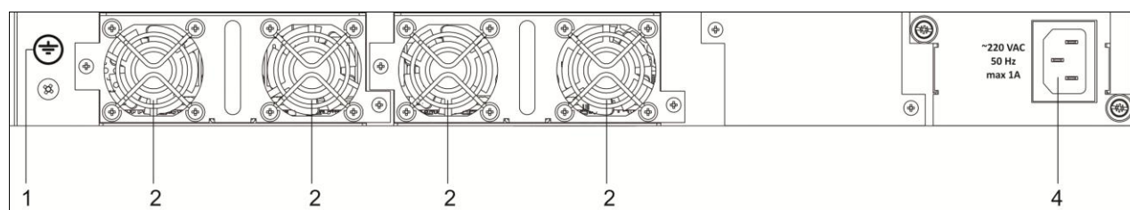
Рисунок 9 – MES5324, задняя панель
