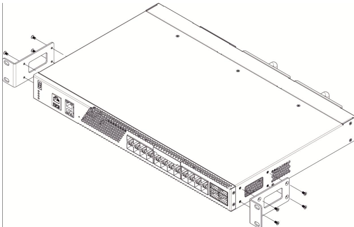
Рисунок 20 – Крепление кронштейнов
