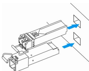
Рисунок 25 – Установка SFP-трансиверов
