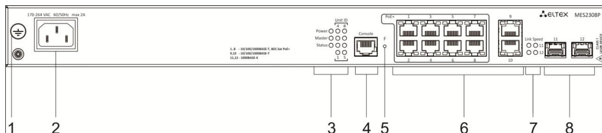
Рисунок 8 – MES2308P, передняя панель
