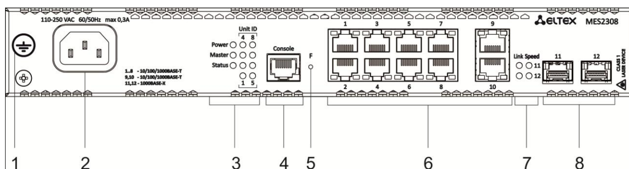
Рисунок 7 – MES2308, передняя панель
