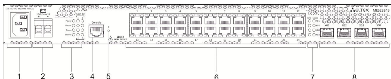
Рисунок 4 – MES2324B, передняя панель
