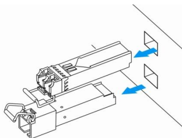
Рисунок 28 – Извлечение SFP-трансиверов
