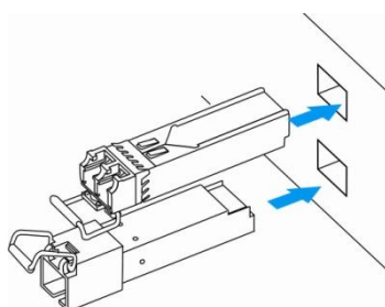
Рисунок 25 – Установка SFP-трансиверов
