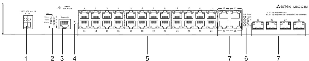
Рисунок 10 – MES1124M DC, передняя панель
