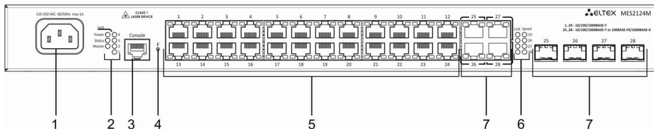
Рисунок 9 – MES2124M AC, передняя панель
