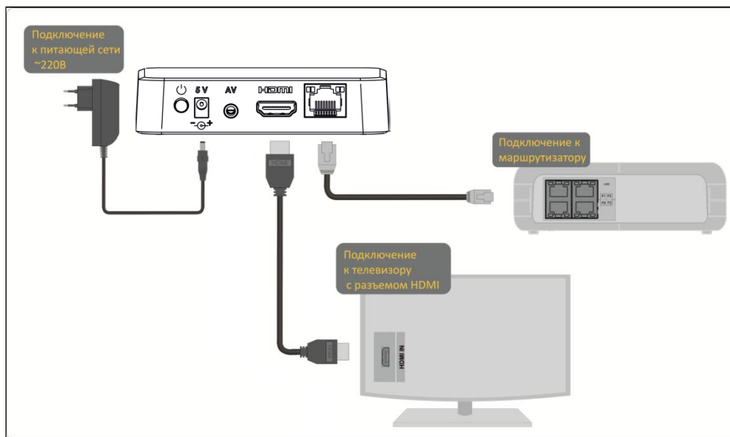
Рисунок 13 — Пример подключения Смарт ТВ-приставки
