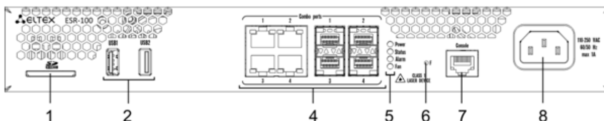
Рисунок 32 – Передняя панель ESR-100
