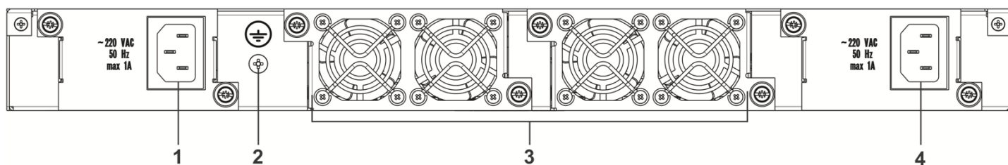
Рисунок 23 – Задняя панель ESR-1511, ESR-1500
