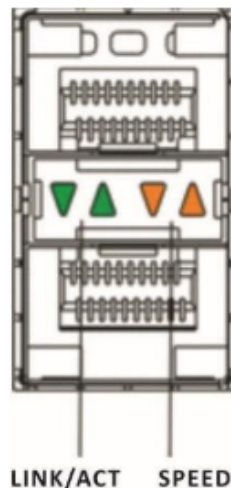
Рисунок 73 – Расположение индикаторов состояния SFP/SFP+/SFP28-интерфейсов
