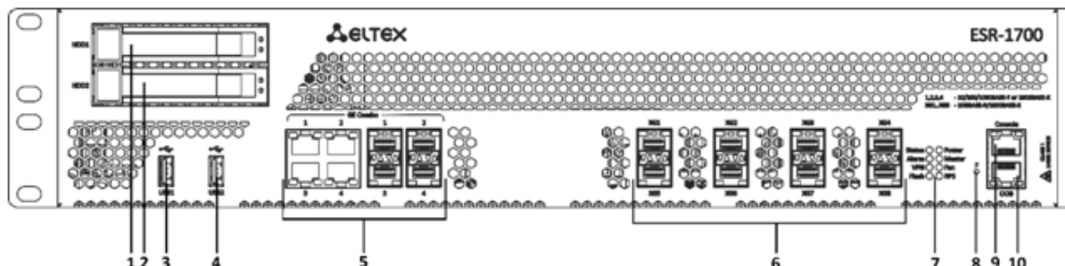
Рисунок 17 – Передняя панель ESR-1700
