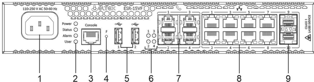
Рисунок 49 – Передняя панель ESR-15VF
