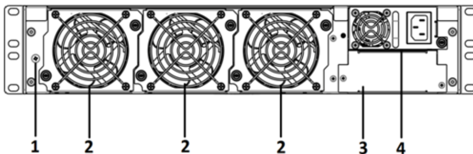
Рисунок 18 – Задняя панель ESR-1700
