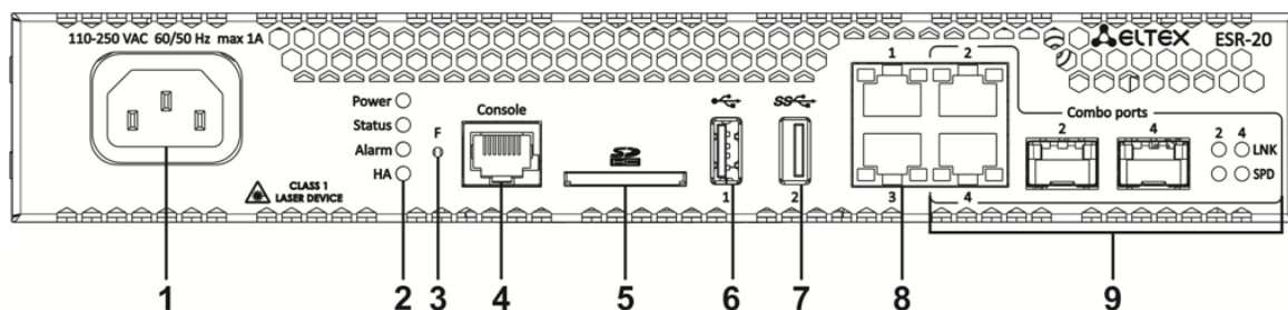
Рисунок 45 – Передняя панель ESR-20
