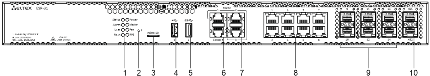
Рисунок 36 – Передняя панель ESR-31
