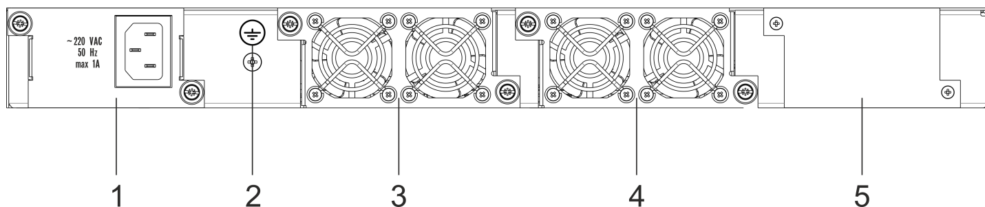
Рисунок 14 – Задняя панель ESR-3100
