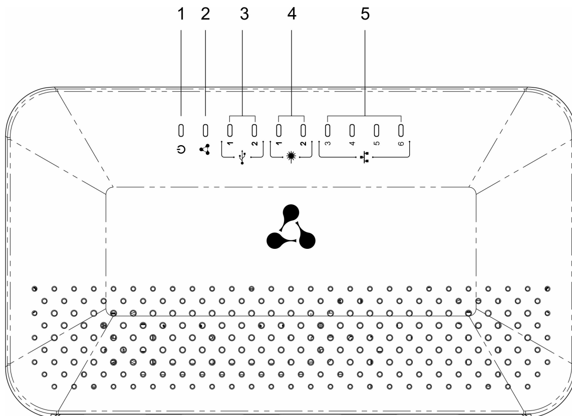
Рисунок 58 – Верхняя панель ESR-15
