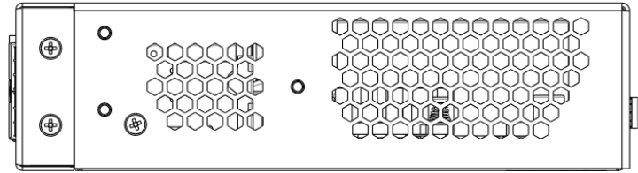
Рисунок 52 – Правая панель ESR-15VF
