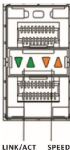
Рисунок 71 – Расположение индикаторов SFP/SFP+/SFP28-интерфейсов
