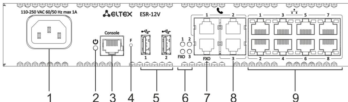
Рисунок 63 – Передняя панель ESR-12V
