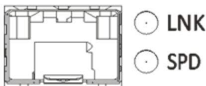
Рисунок 78 – Расположение индикаторов состояния SFP/SFP+-интерфейсов
