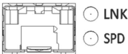
Рисунок 83 – Расположение индикаторов разъема SFP
