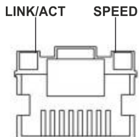
Рисунок 84 – Расположение индикаторов разъема RJ-45
