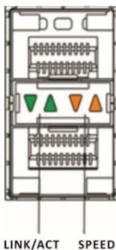
Рисунок 75 – Расположение индикаторов состояния SFP/SFP+-интерфейсов
