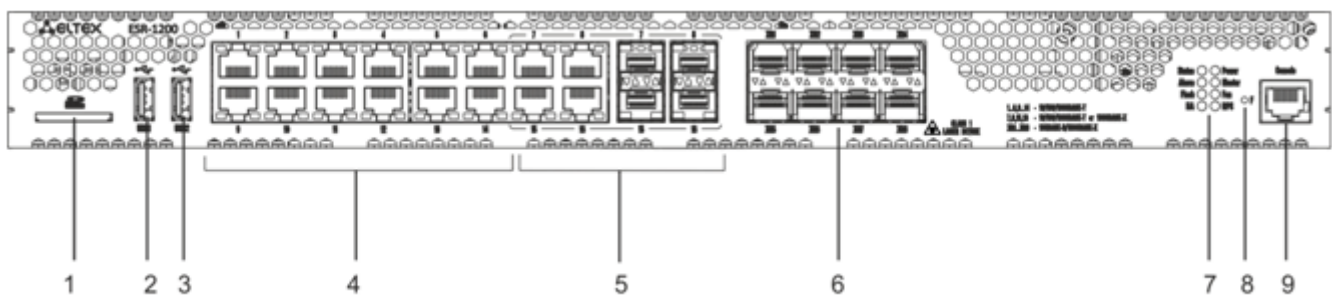
Рисунок 26 – Передняя панель ESR-1200
