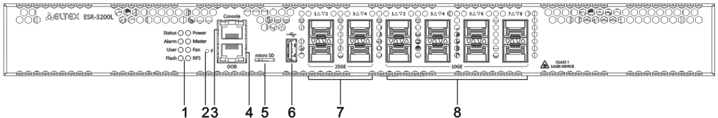
Рисунок 5 – Передняя панель ESR-3200L
