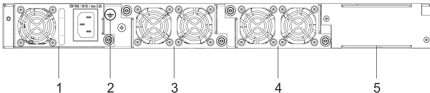
Рисунок 10 – Задняя панель ESR-3200
