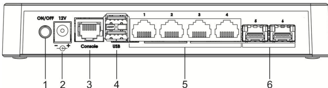
Рисунок 67 – Задняя панель ESR-10
