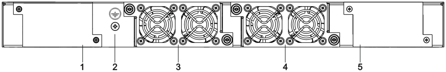
Рисунок 6 – Задняя панель ESR-3200L
