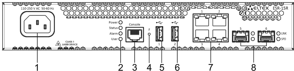
Рисунок 53 – Передняя панель ESR-15R
