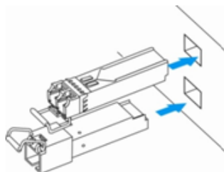
Рисунок 94 – Установка SFP-трансиверов
