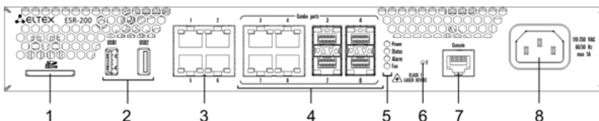
Рисунок 31 – Передняя панель ESR-200
