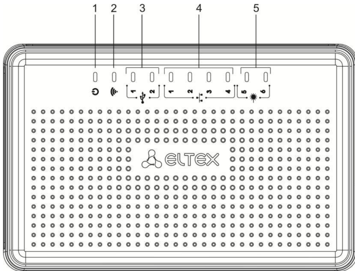
Рисунок 69 – Верхняя панель маршрутизатора ESR-10
