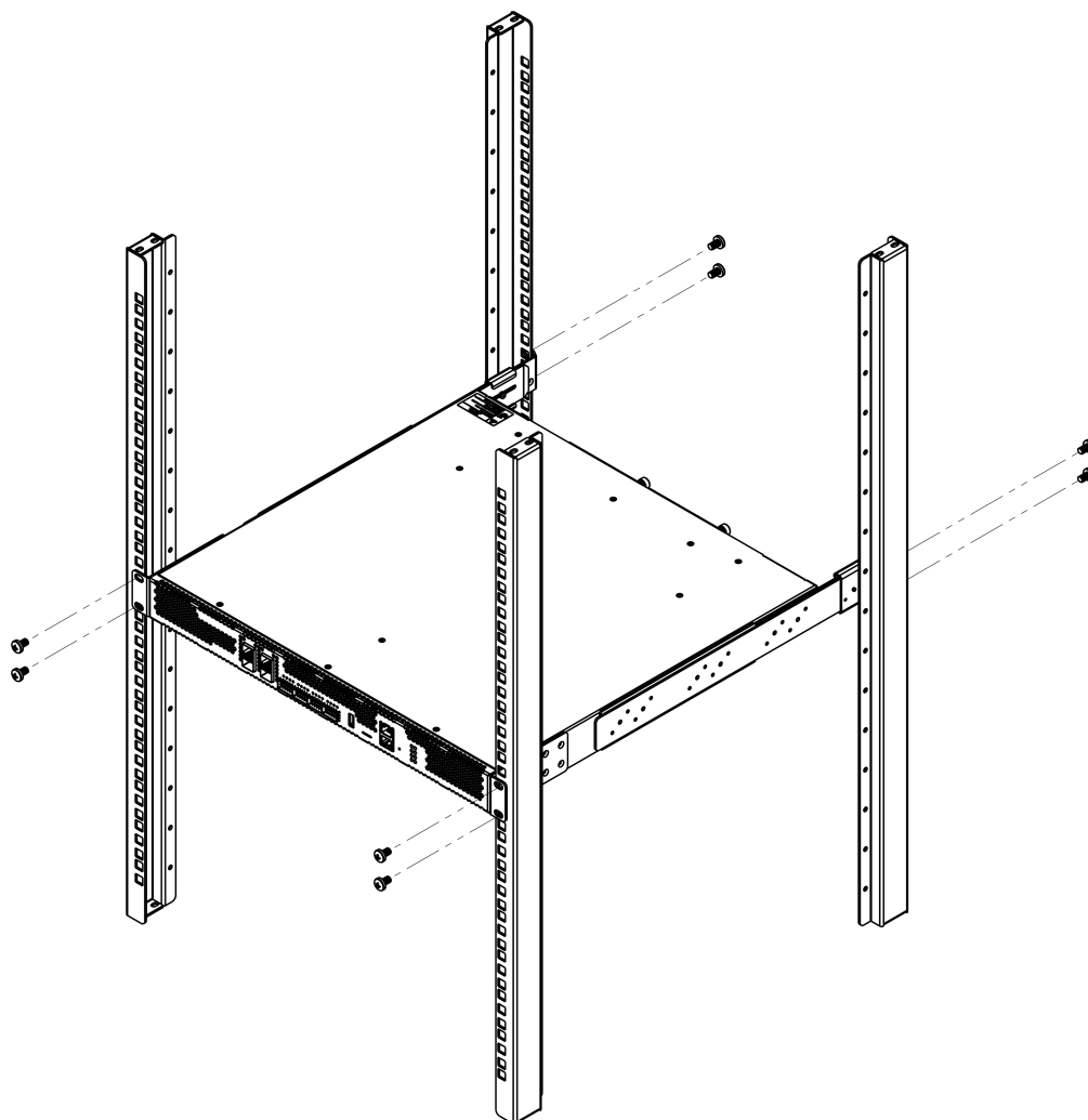
Рисунок 91 – Установка ESR-3300 в стойку
