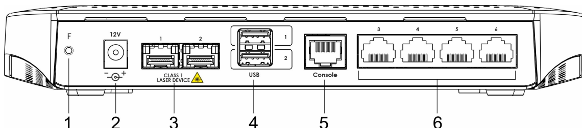
Рисунок 57 – Задняя панель ESR-15
