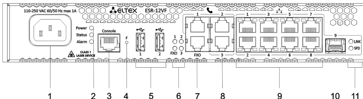
Рисунок 59 – Передняя панель ESR-12VF
