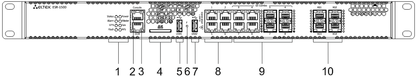
Рисунок 22 – Передняя панель ESR-1500
