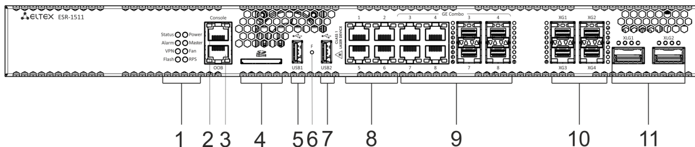
Рисунок 21 – Передняя панель ESR-1511
