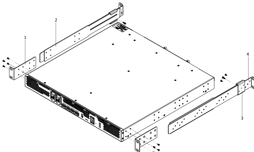
Рисунок 90 – Крепление кронштейнов к ESR-3300
