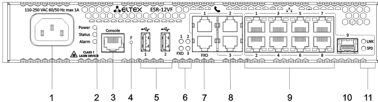
Рисунок 59 – Передняя панель ESR-12VF
