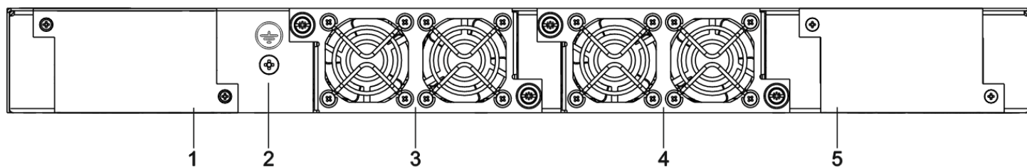
Рисунок 6 – Задняя панель ESR-3200L
