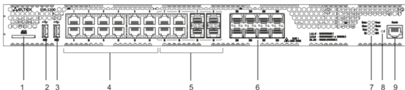
Рисунок 26 – Передняя панель ESR-1200
