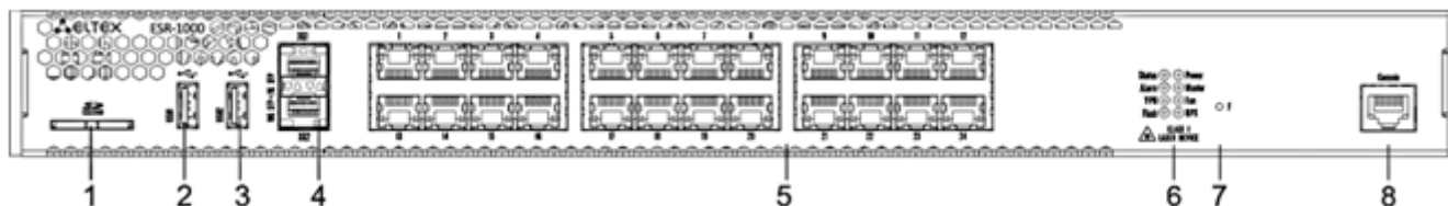
Рисунок 27 – Передняя панель ESR-1000
