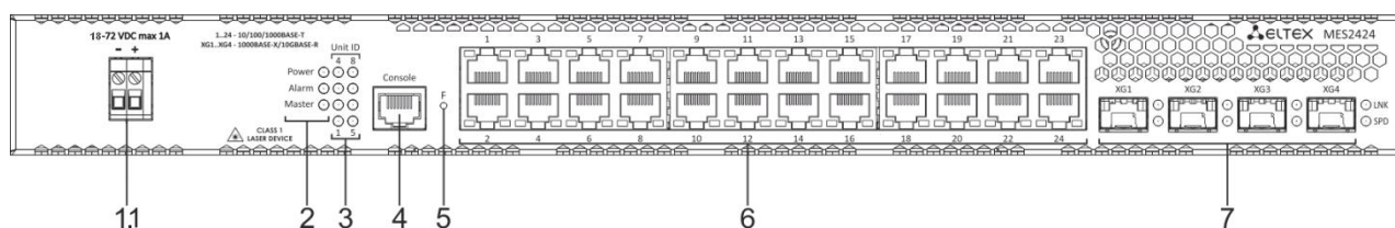
Рисунок 18 – Передняя панель MES2424 DC
