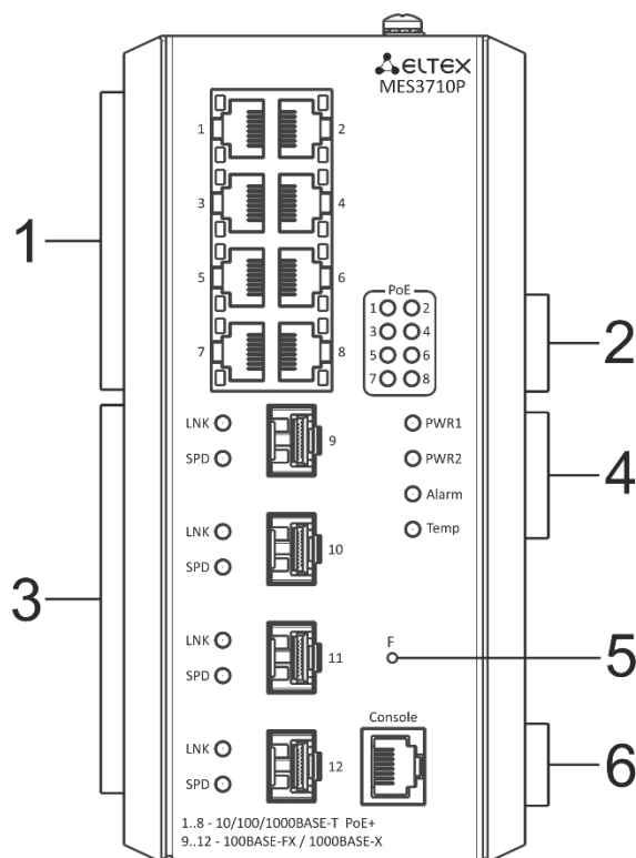
Рисунок 35 – Передняя панель MES3710P
