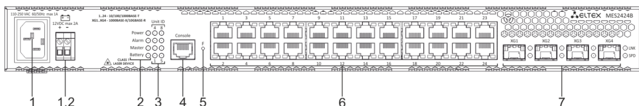
Рисунок 19 – Передняя панель MES2424B
