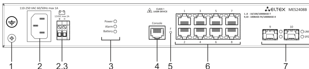
Рисунок 5 – Передняя панель MES2408B
