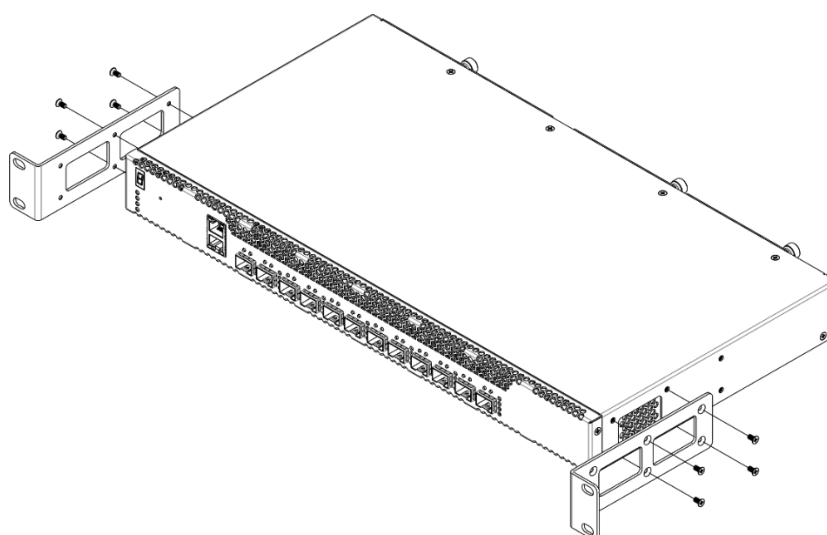
Рисунок 56 – Вариант крепления кронштейнов №2
