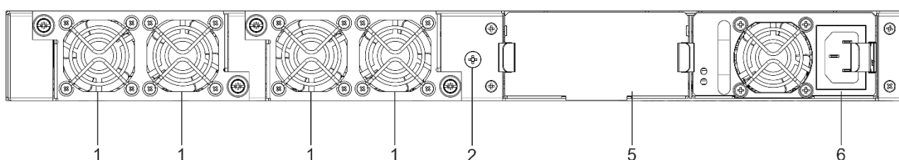
Рисунок 42 – Задняя панель MES2420-48P
