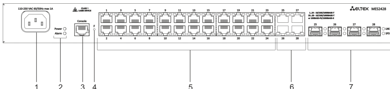
Рисунок 12 – Передняя панель MES2428 AC
