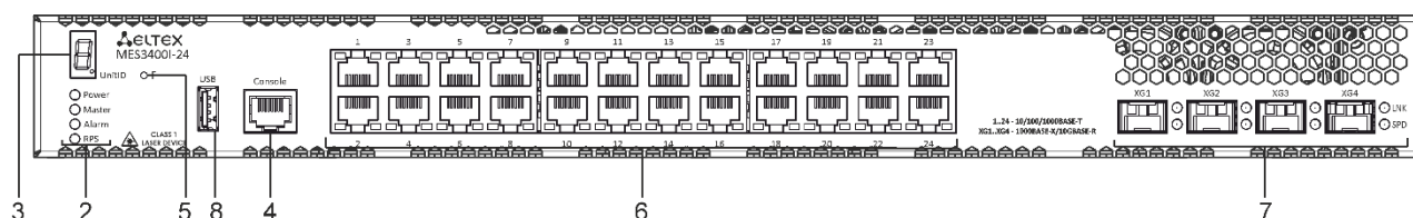
Рисунок 27 – Передняя панель MES3400I-24
