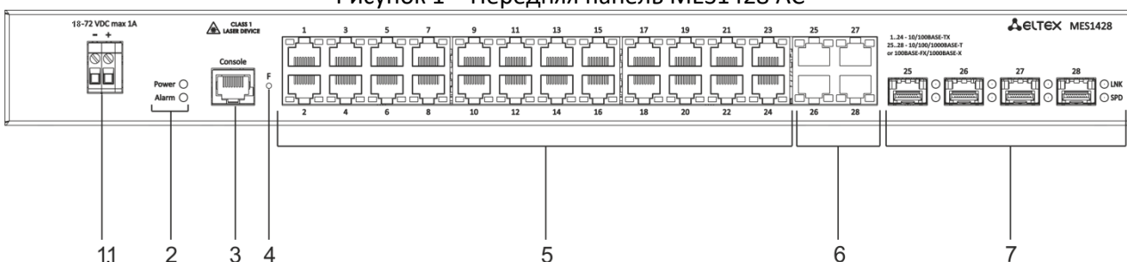
Рисунок 2 – Передняя панель MES1428 DC
