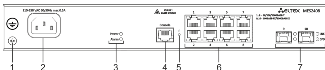
Рисунок 3 – Передняя панель MES2408 AC
