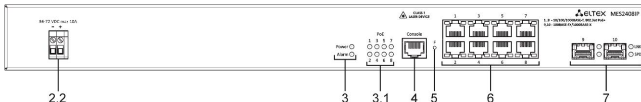
Рисунок 8 – Передняя панель MES2408IP DC1
