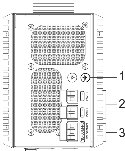
Рисунок 48 — Верхняя панель MES3710P
