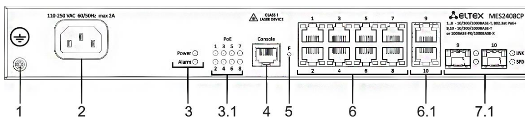
Рисунок 7 – Передняя панель MES2408CP
