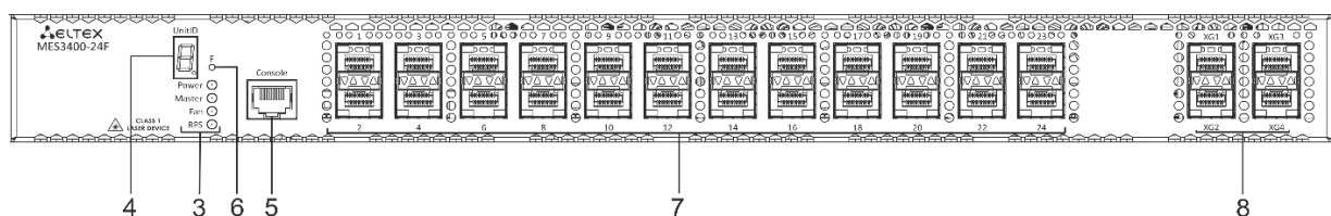
Рисунок 30 – Передняя панель MES3400-24F
