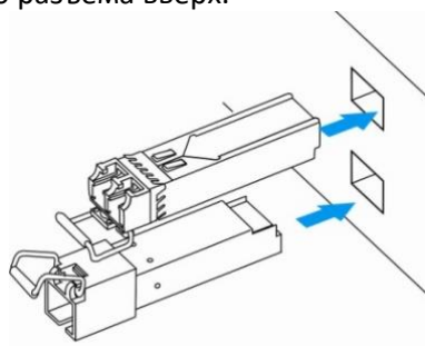
Рисунок 59 – Установка SFP-трансиверов
