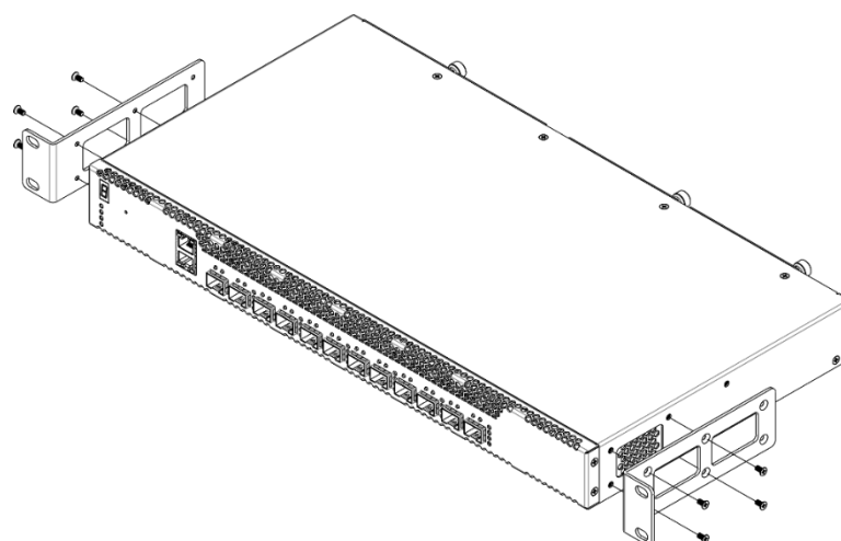
Рисунок 55 – Вариант крепления кронштейнов №1
