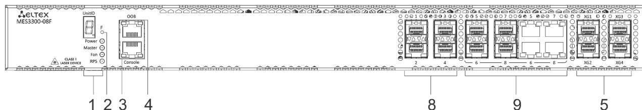
Рисунок 13 – Передняя панель MES3300-08F
