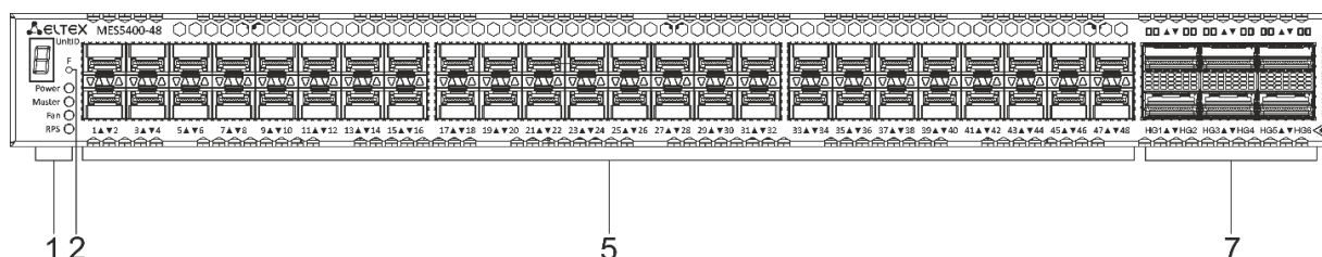
Рисунок 24 – Передняя панель MES5400-48
