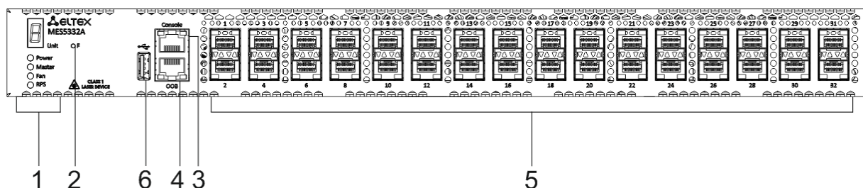
Рисунок 21 – Передняя панель MES5332A
