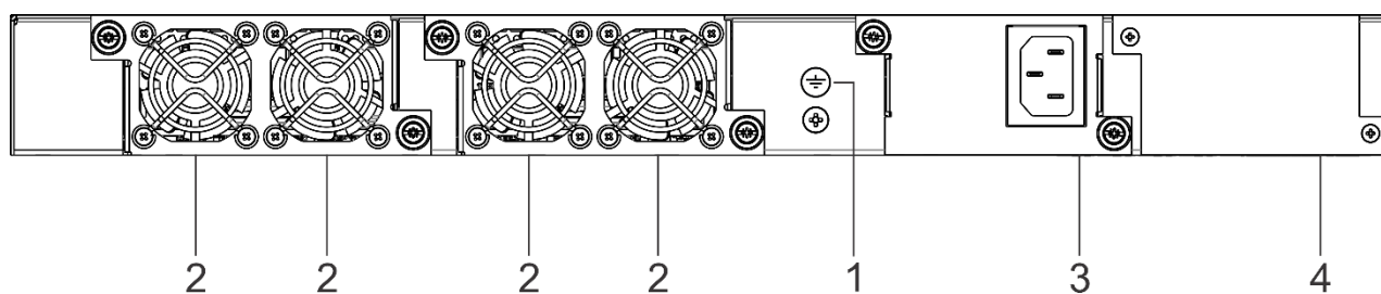
Рисунок 40 – Задняя панель MES3300-24F
