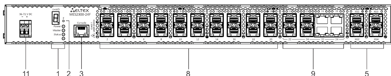
Рисунок 4 – Передняя панель MES2300-24F
