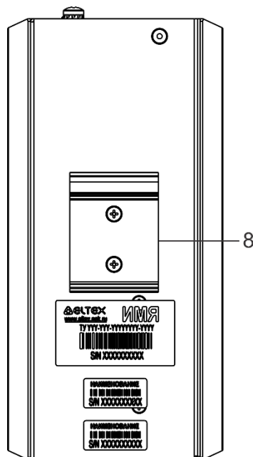
Рисунок 42 – Задняя панель MES3500I-08P, MES3500I-10P
