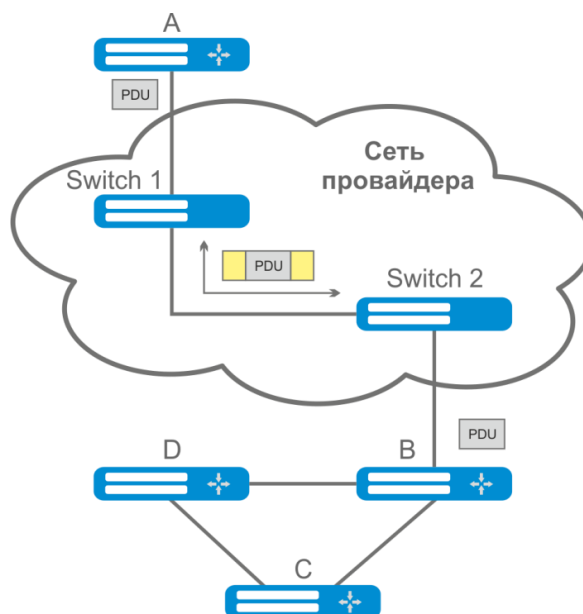
Рисунок 88 — Пример работы функции L2PT
