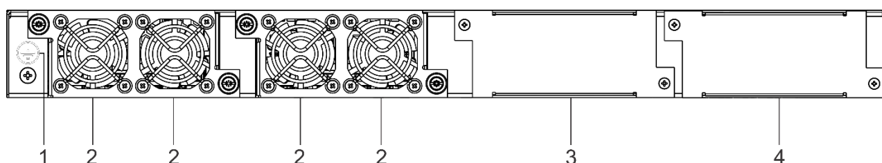
Рисунок 33 – Задняя панель MES2300D-24P
