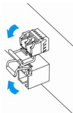
Рисунок 85 – Открытие защелки SFP-трансиверов
