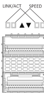
Рисунок 74 – Внешний вид разъема QSFP+ и QSFP28 для MES5400-xx, MES5410-48
