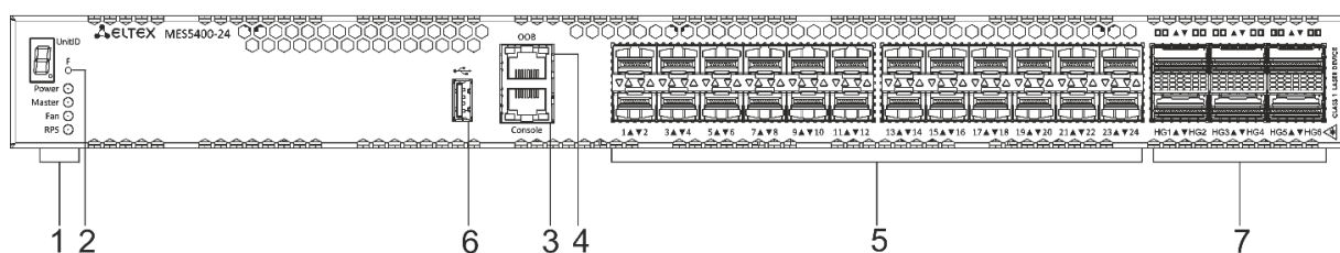
Рисунок 23 – Передняя панель MES5400-24
