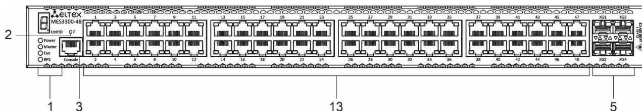
Рисунок 16 – Передняя панель MES3300-48
