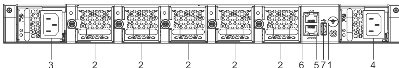
Рисунок 48 – Задняя панель MES5410-48
