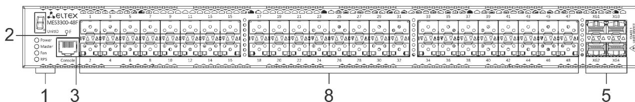
Рисунок 17 – Передняя панель MES3300-48F
