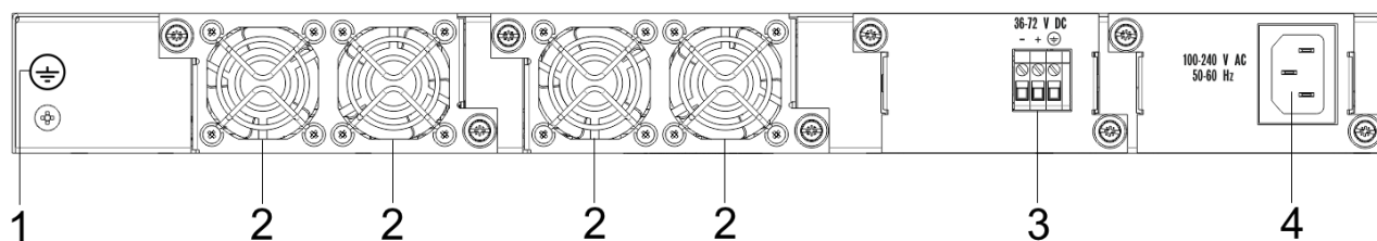
Рисунок 43 – Задняя панель MES5312, MES5324A, MES5332A
