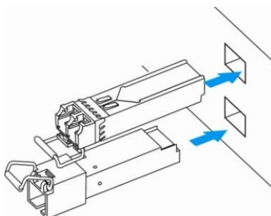
Рисунок 83 – Установка SFP-трансиверов
