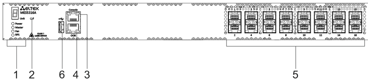
Рисунок 19 – Передняя панель MES5316A
