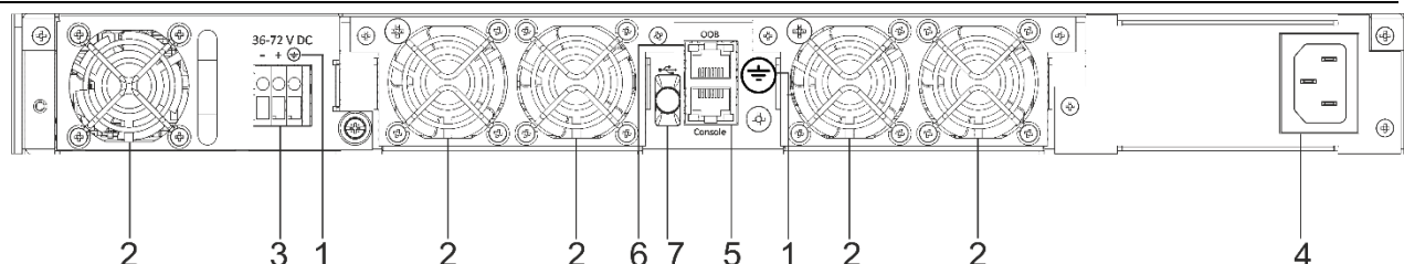
Рисунок 47 – Задняя панель MES5400-48
