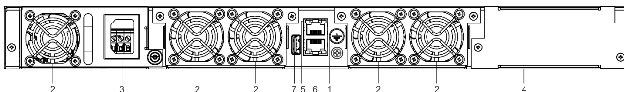
Рисунок 45 – Задняя панель MES5310-48
