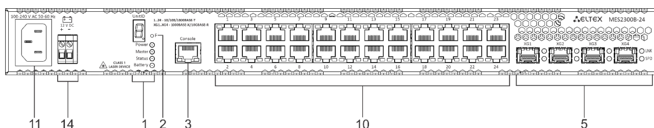
Рисунок 3 – Передняя панель MES2300B-24
