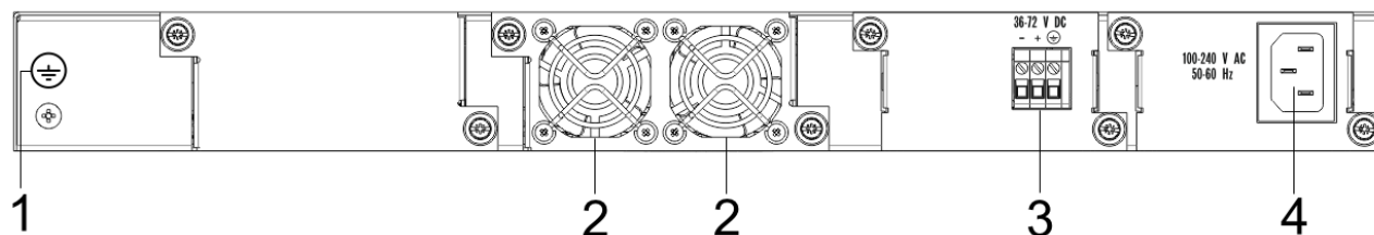
Рисунок 44 – Задняя панель MES5316A
