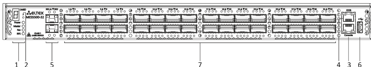
Рисунок 26 – Передняя панель MES5500-32
