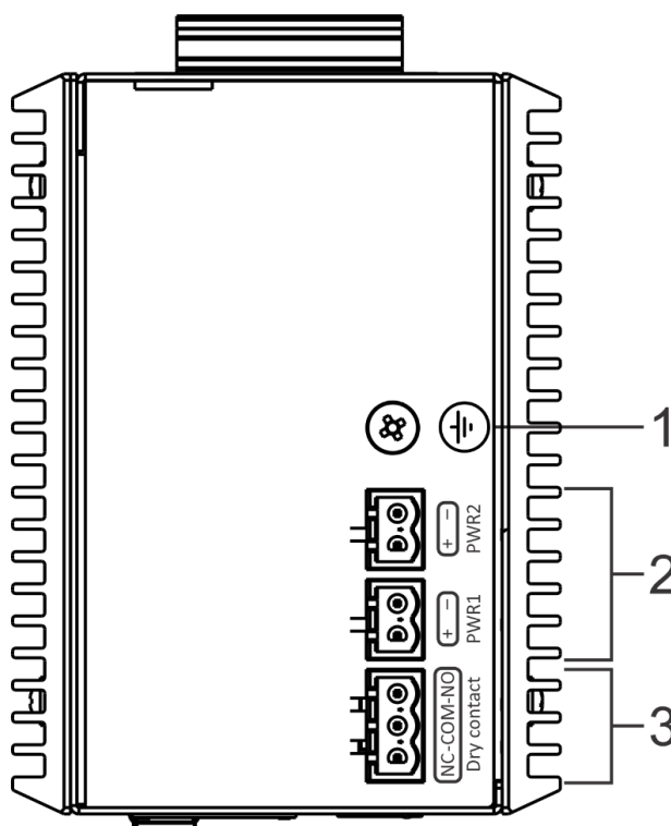
Рисунок 29 – Верхняя панель MES3500I-08P и MES3500I-10P
