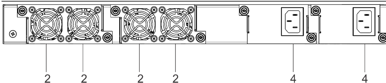
Рисунок 37 – Задняя панель MES3300-24
