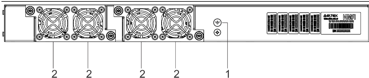
Рисунок 31 – Задняя панель MES2300-24F, MES2300B-24F
