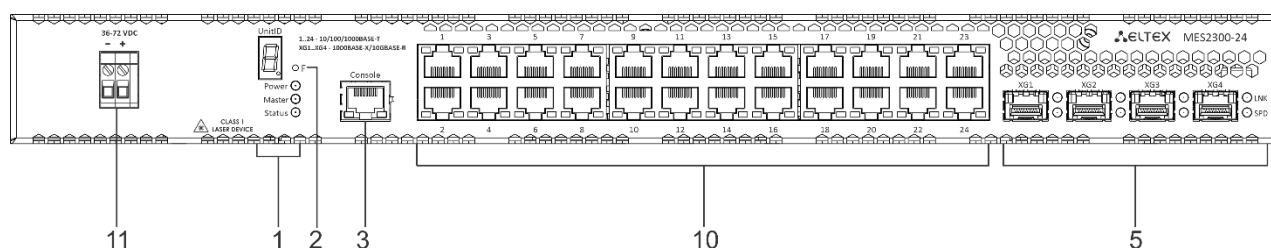
Рисунок 2 – Передняя панель MES2300-24 DC
