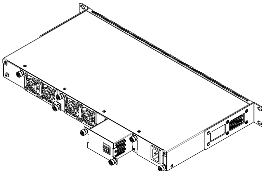
Рисунок 82 – Установка модулей питания
