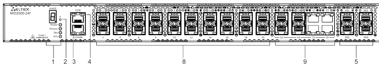
Рисунок 15 – Передняя панель MES3300-24F
