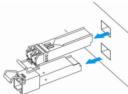
Рисунок 86 – Извлечение SFP-трансиверов
