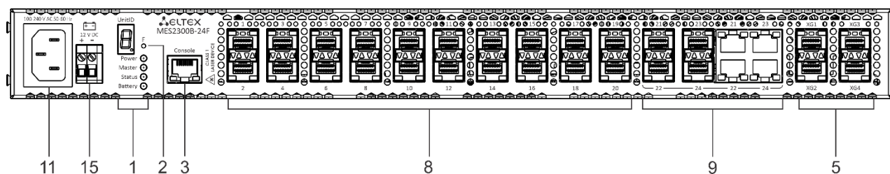
Рисунок 7 – Передняя панель MES2300B-24F
