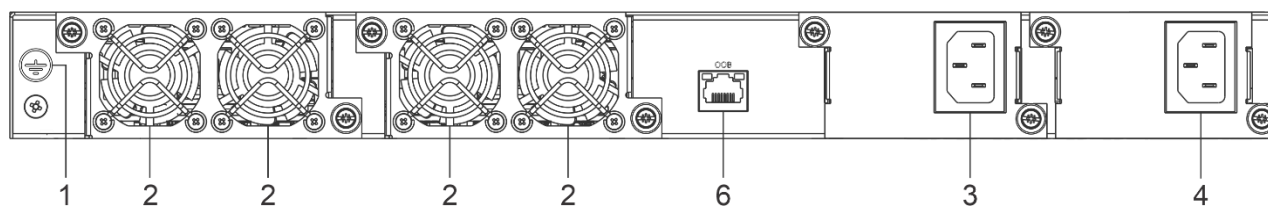
Рисунок 41 – Задняя панель MES3300-48, MES3300-48F
