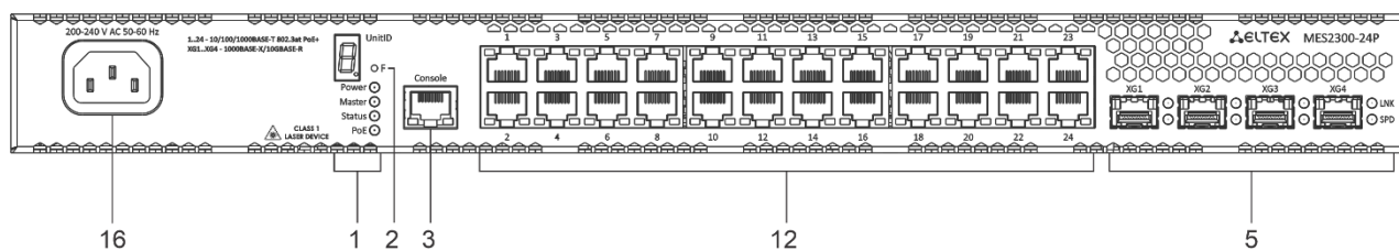
Рисунок 8 – Передняя панель MES2300-24P
