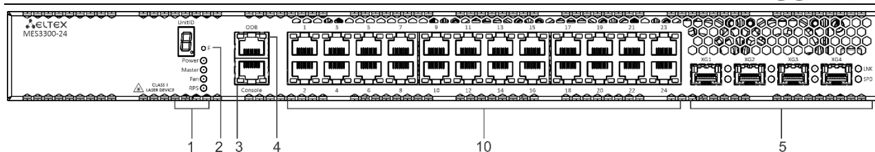
Рисунок 12 – Передняя панель MES3300-24
