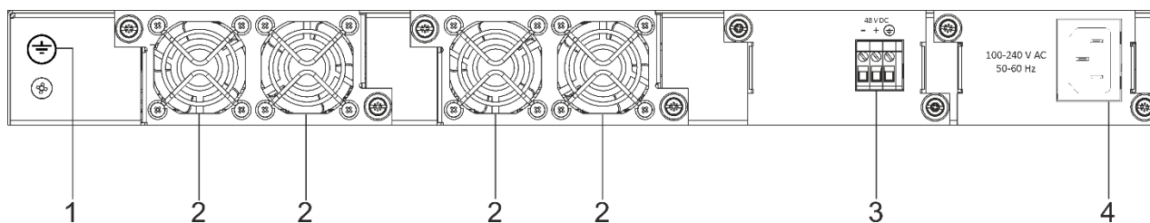
Рисунок 46 – Задняя панель MES5400-24
