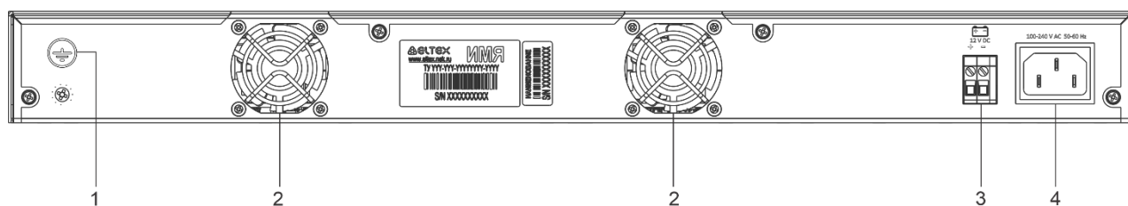
Рисунок 36 – Задняя панель MES2300B-48
