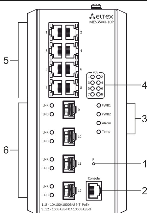
Рисунок 28 – Передняя панель MES3500I-10P
