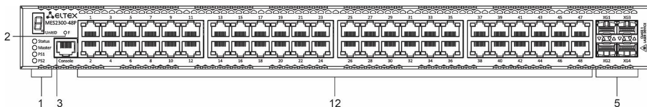
Рисунок 10 – Передняя панель MES2300-48P
