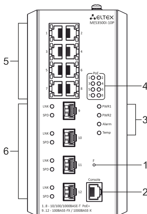
Рисунок 27 – Передняя панель MES3500I-08P
