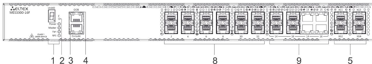
Рисунок 14 – Передняя панель MES3300-16F
