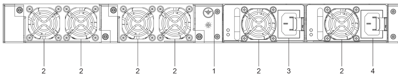
Рисунок 35 – Задняя панель MES2300-48P
