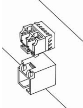
Рисунок 84 – Установленные SFP-трансиверы
