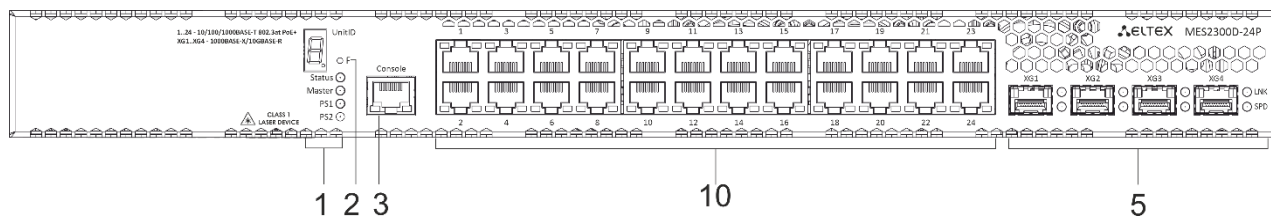
Рисунок 9 – Передняя панель MES2300D-24P
