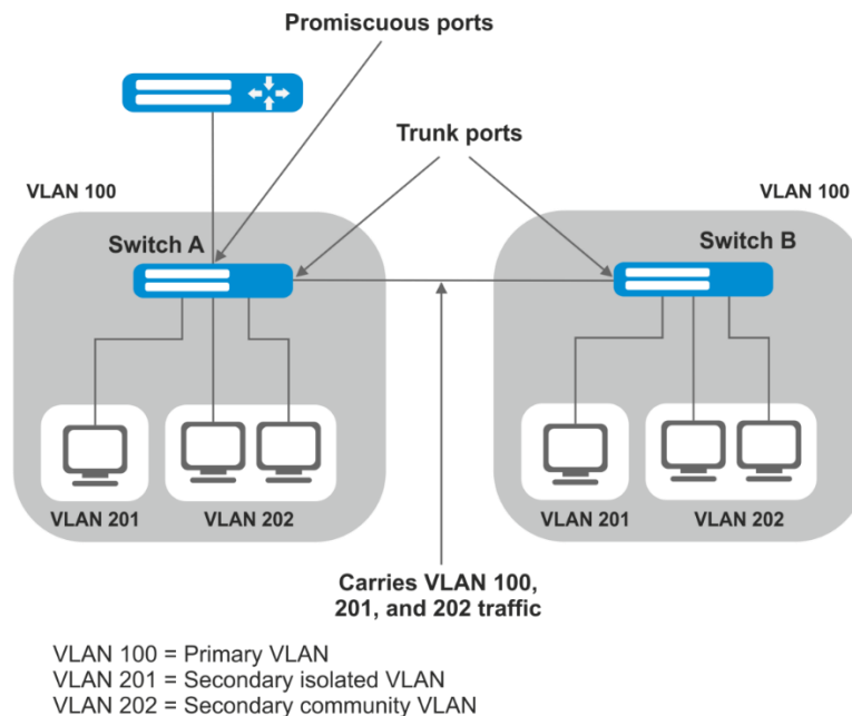
Рисунок 87 – Пример работы технологии Private VLAN
