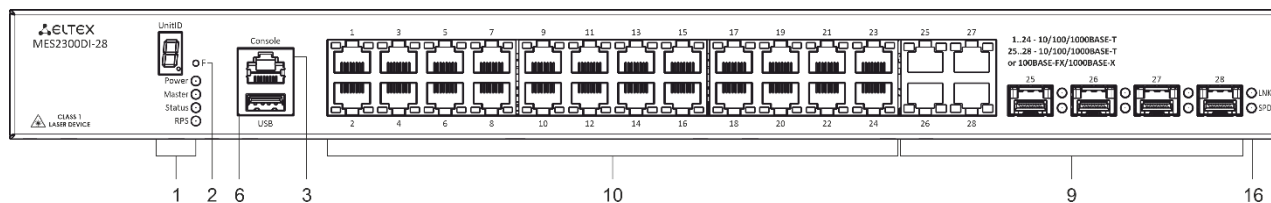
Рисунок 6 – Передняя панель MES2300DI-28
