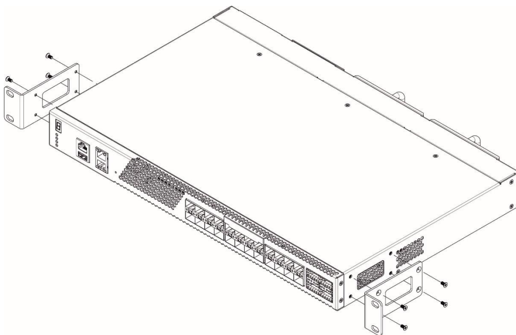
Рисунок 42 — Крепление кронштейнов
