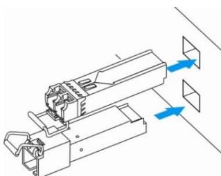
Рисунок 47 — Установка SFP-трансиверов
