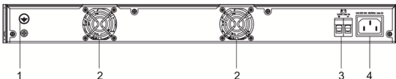
Рисунок 32 — Задняя панель MES2348B
