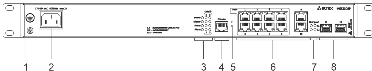
Рисунок 17 — Передняя панель MES2308P
