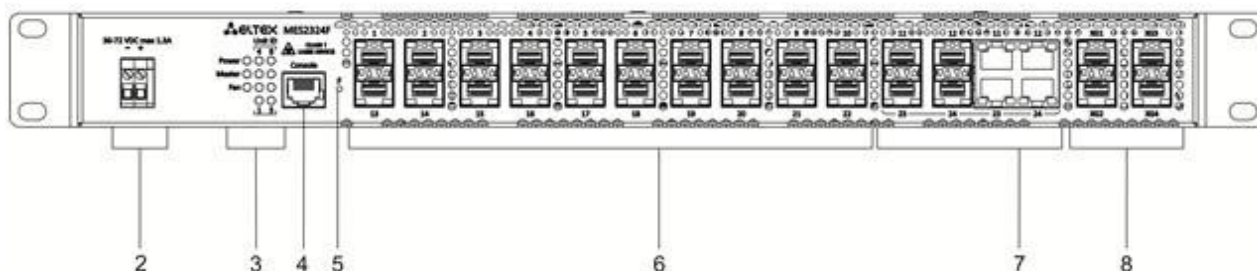
Рисунок 11 — Передняя панель MES2324F DC
