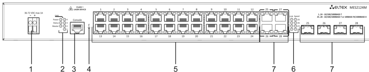
Рисунок 10 – MES1124M DC, передняя панель
