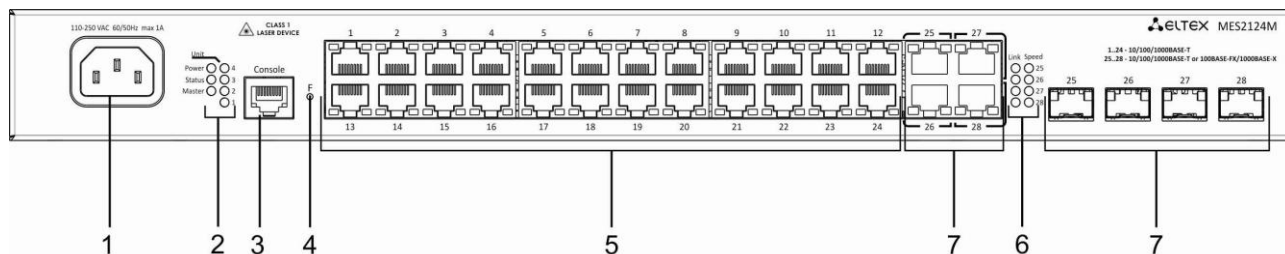
Рисунок 9 – MES2124M AC, передняя панель
