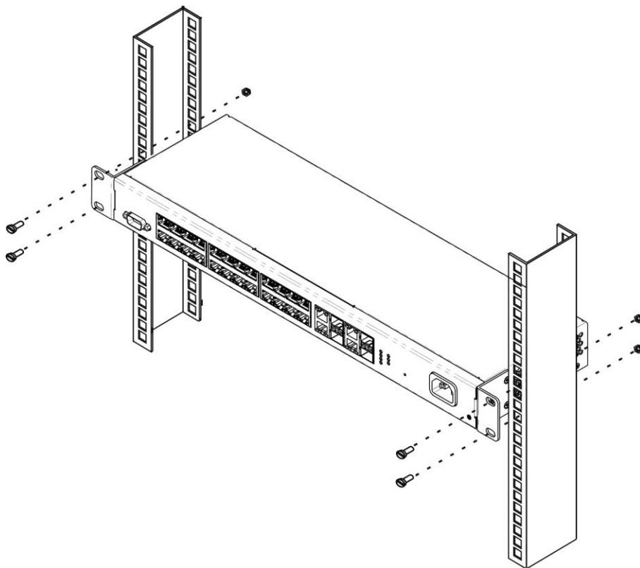
Рисунок 22 – Установка устройства в стойку
