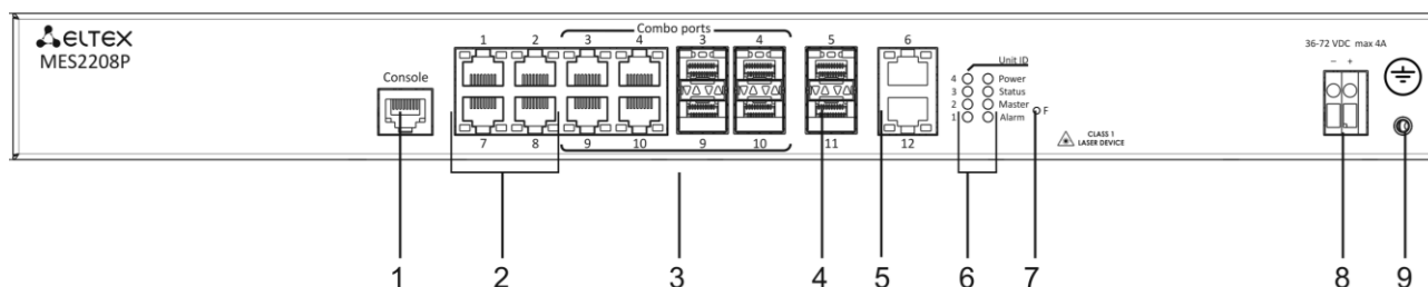
Рисунок 12 – MES2208P, передняя панель
