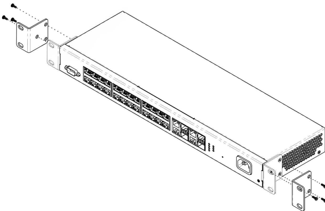
Рисунок 21 – Крепление кронштейнов
