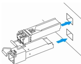
Рисунок 25 – Установка SFP-трансиверов
