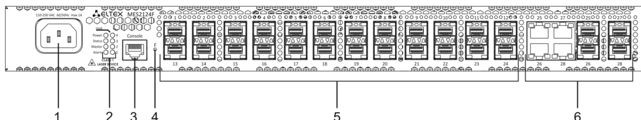
Рисунок 15 – MES2124F, передняя панель
