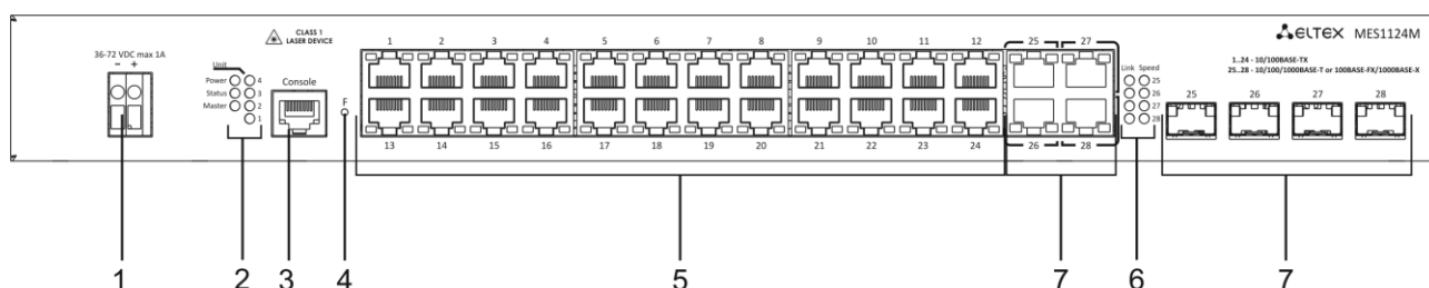
Рисунок 8 – MES1124M DC, передняя панель
