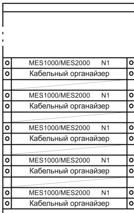
Рисунок 23 – Размещение коммутаторов в стойке
