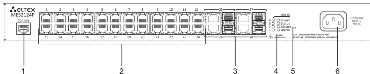
Рисунок 13 – MES2124P, передняя панель
