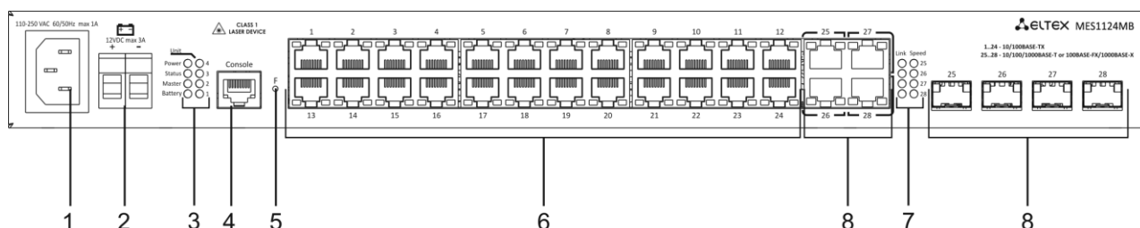
Рисунок 4 – MES1124MB, передняя панель
