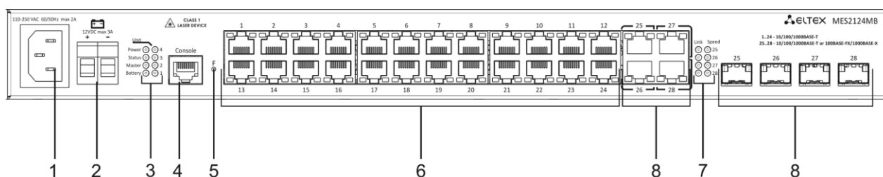
Рисунок 5 – MES2124MB, передняя панель
