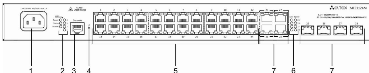
Рисунок 7 – MES1124M AC, передняя панель
