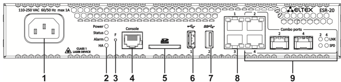
Рисунок 33 – Передняя панель ESR-20
