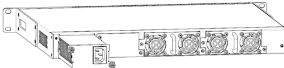
Рисунок 69 – Установка модулей питания
