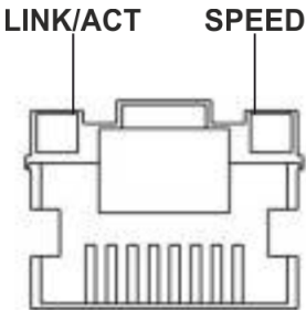
Рисунок 66 – Расположение индикаторов разъема RJ-45
