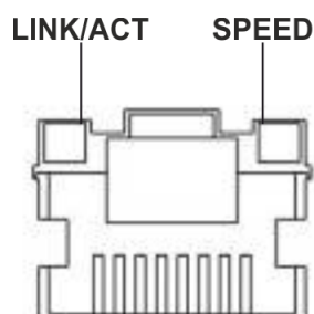
Рисунок 60 – Расположение индикаторов разъема RJ-45
