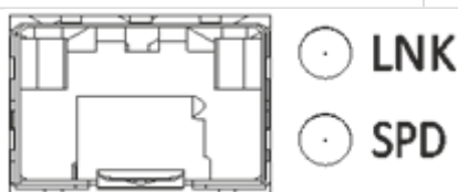
Рисунок 61 – Расположение индикаторов разъема SFP
