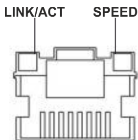
Рисунок 56 – Расположение индикаторов разъема RJ-45
