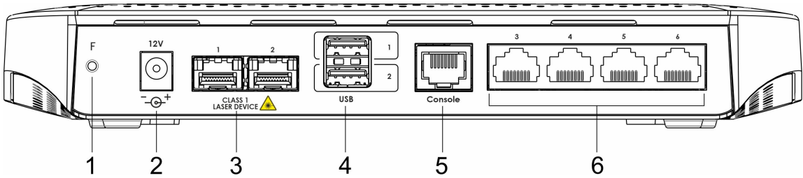
Рисунок 37 – Задняя панель ESR-15
