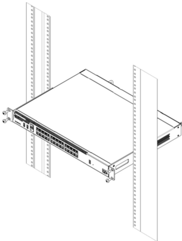
Рисунок 68 – Установка устройства в стойку
