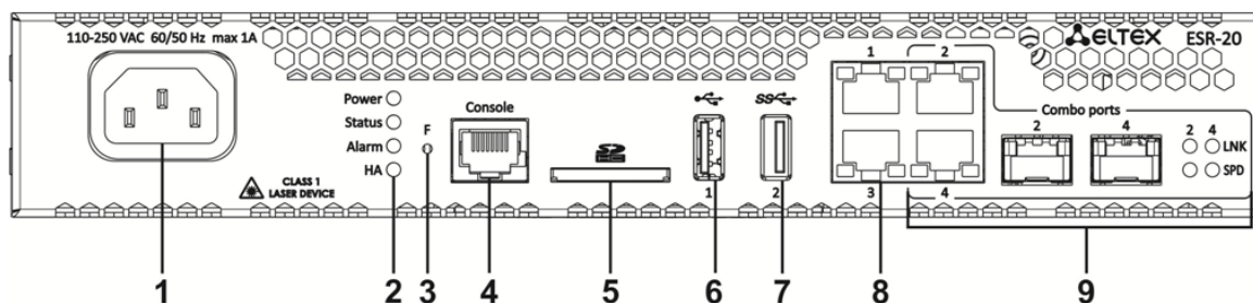
Рисунок 33 – Передняя панель ESR-20
