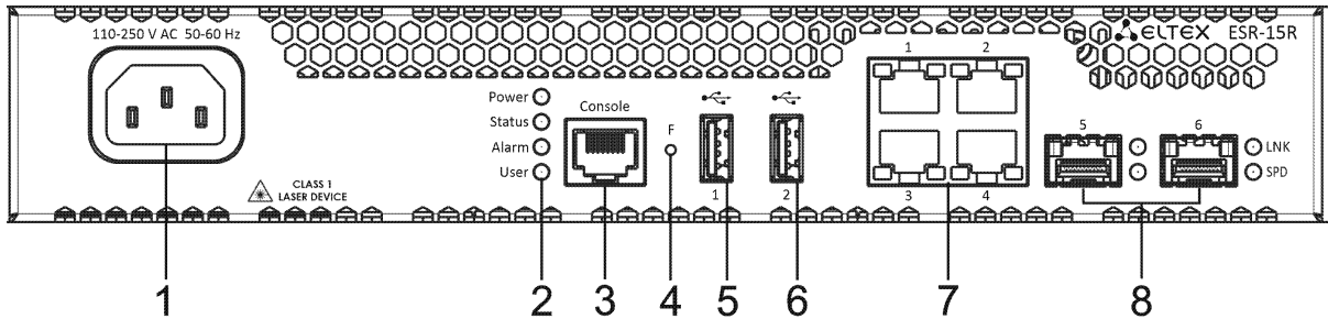
Рисунок 39 – Передняя панель ESR-15R
