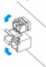
Рисунок 73 – Открытие защелки SFP-трансиверов
