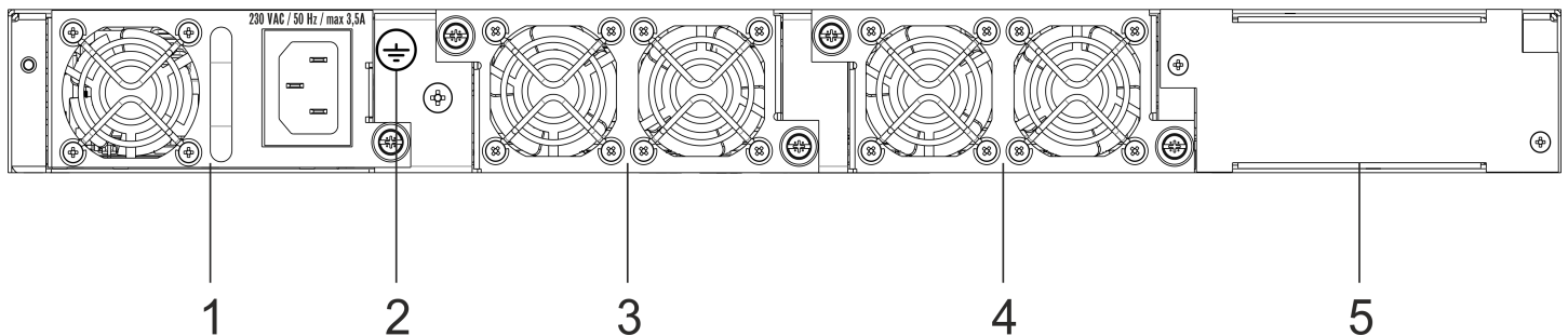
Рисунок 2 – Задняя панель ESR-3200
