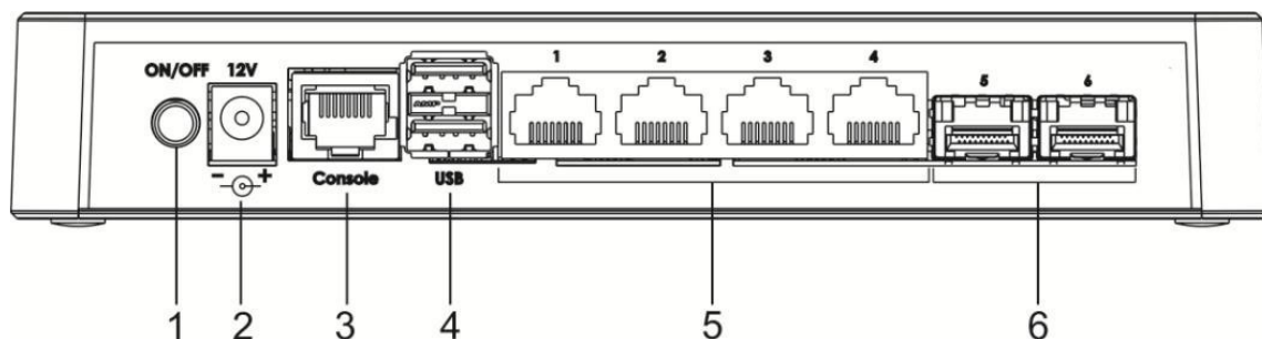
Рисунок 51 – Задняя панель ESR-10
