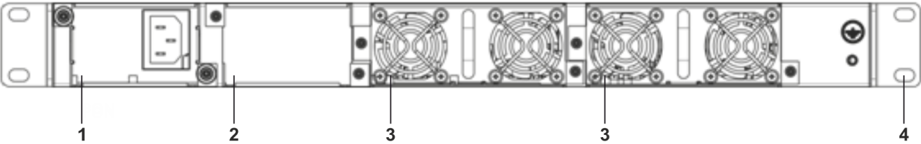
Рисунок 20 – Задняя панель ESR-1000
