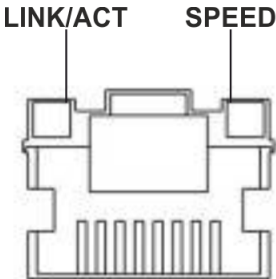
Рисунок 54 – Расположение индикаторов разъема RJ-45
