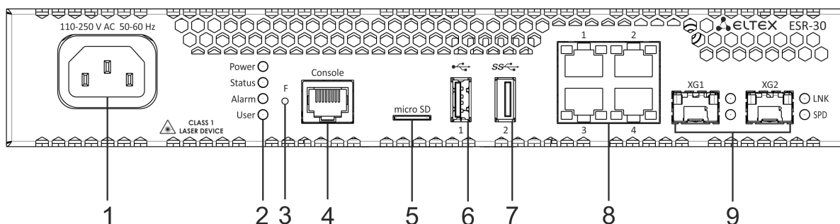
Рисунок 32 – Передняя панель ESR-30
