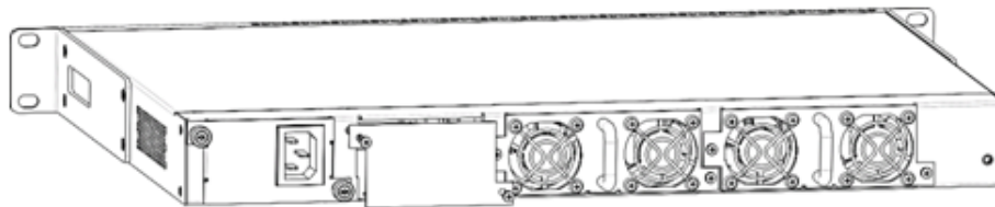
Рисунок 70 – Установка заглушки
