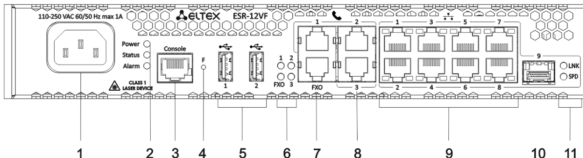
Рисунок 43 – Передняя панель ESR-14VF, ESR-12VF
