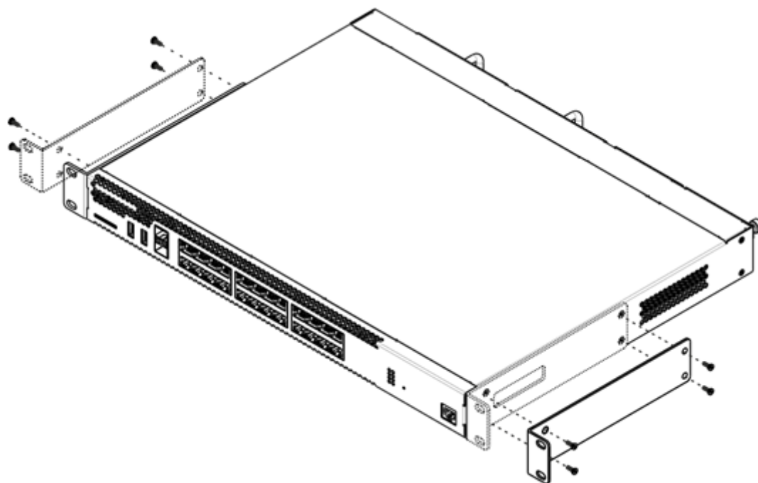
Рисунок 67 – Крепление кронштейнов
