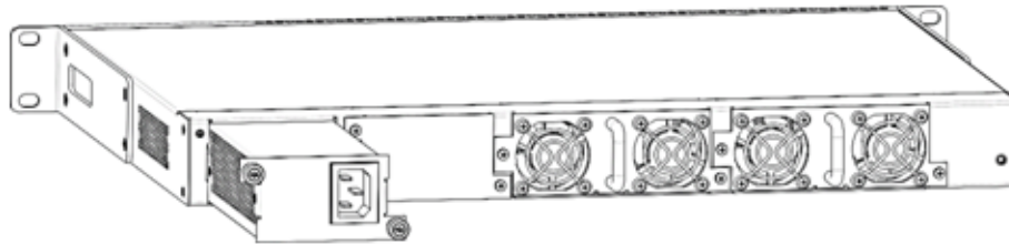
Рисунок 69 – Установка модулей питания
