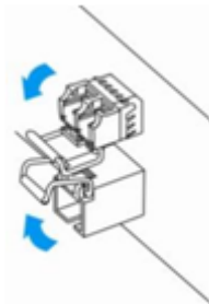
Рисунок 41 – Открытие защелки SFP-трансиверов
