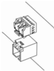
Рисунок 40 – Установленные SFP-трансиверы
