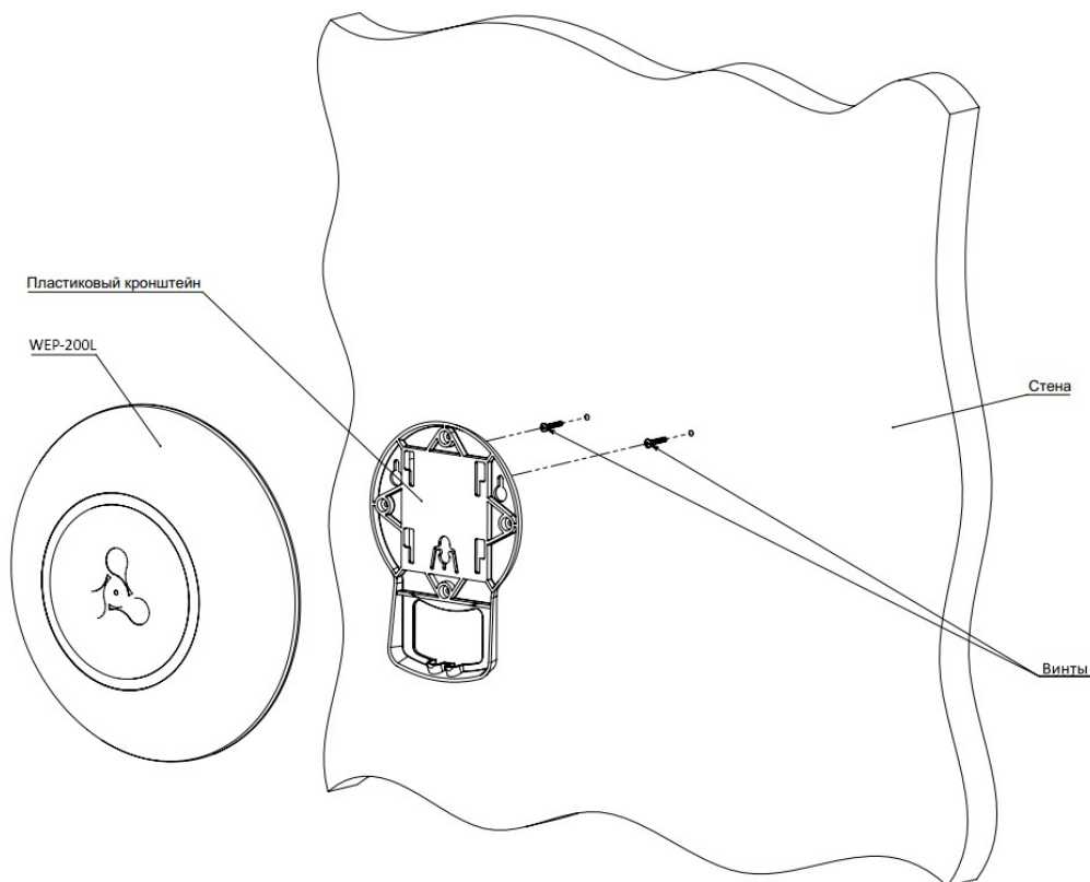
Рисунок 8 – Крепление кронштейна на стене
