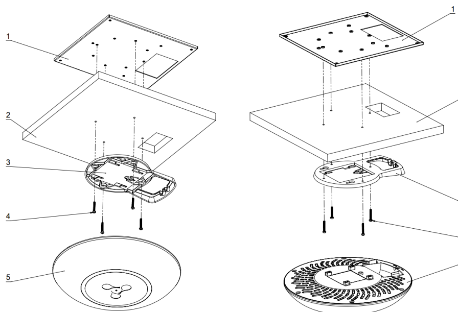
Рисунок 9 — Монтаж устройства на фальшпотолок
