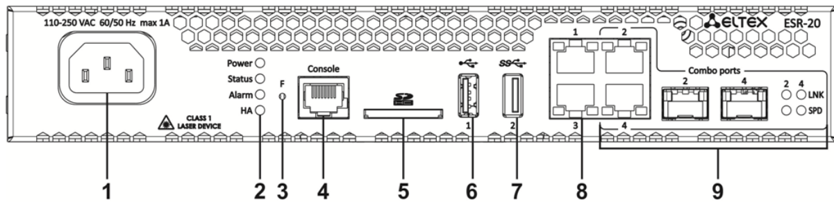
Рисунок 24 – Передняя панель ESR-20
