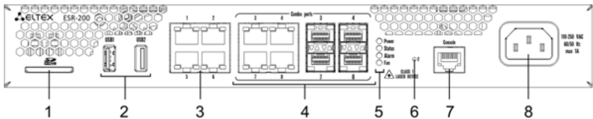
Рисунок 14 – Передняя панель ESR-200
