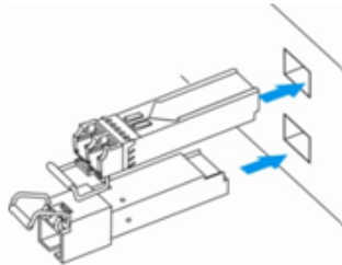
Рисунок 39 – Установка SFP-трансиверов
