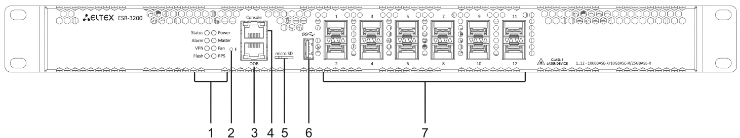
Рисунок 1 – Передняя панель ESR-3200
