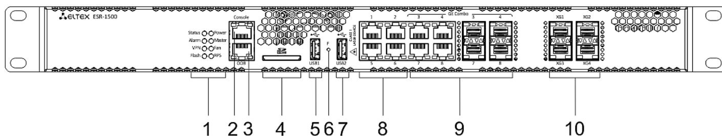
Рисунок 6 – Передняя панель ESR-1500
