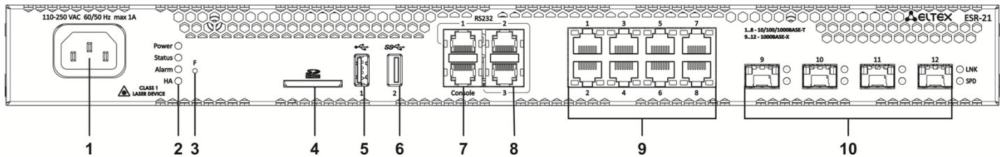
Рисунок 19 – Передняя панель ESR-21
