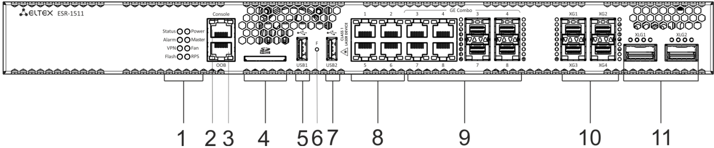
Рисунок 5 – Передняя панель ESR-1511
