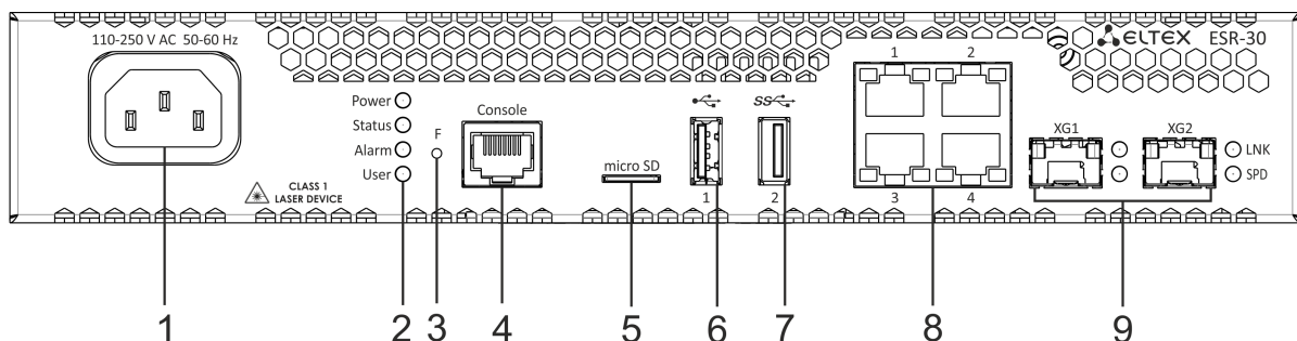
Рисунок 23 – Передняя панель ESR-30
