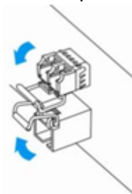
Рисунок 41 – Открытие защелки SFP-трансиверов
