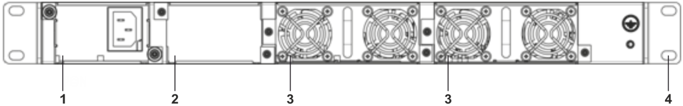
Рисунок 11 – Задняя панель ESR-1000
