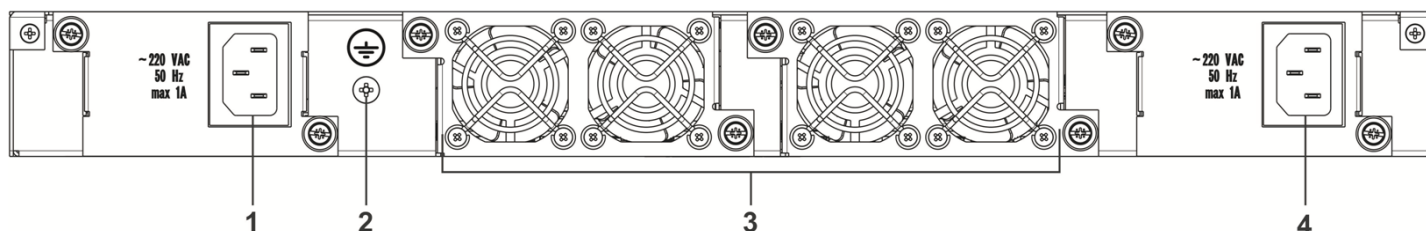
Рисунок 7 – Задняя панель ESR-1511, ESR-1500
