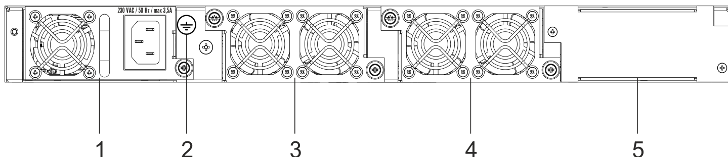
Рисунок 2 – Задняя панель ESR-3200
