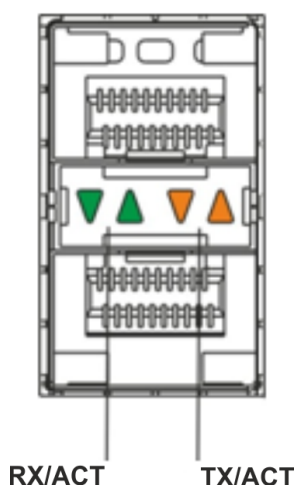
Рисунок 31 – Расположение индикаторов оптических интерфейсов
