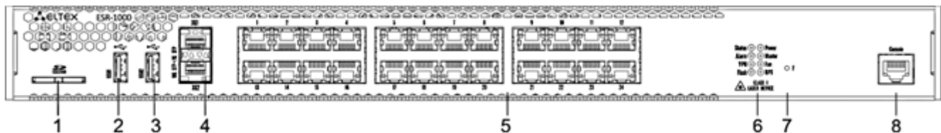
Рисунок 10 – Передняя панель ESR-1000
