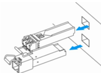
Рисунок 42 – Извлечение SFP-трансиверов
