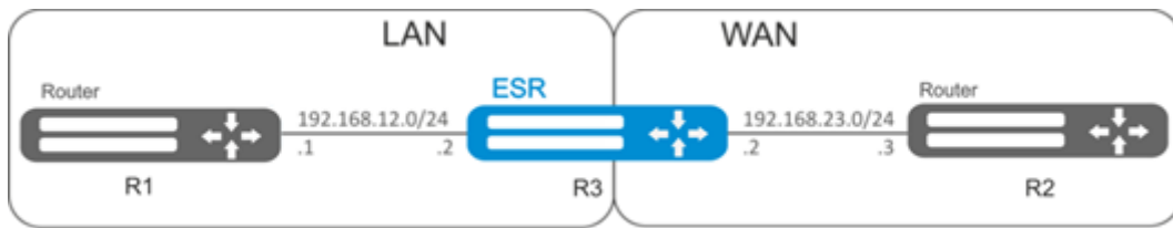
Рисунок 37 – Схема сети
