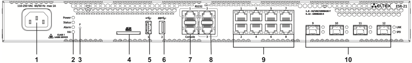
Рисунок 32 – Передняя панель ESR-21
