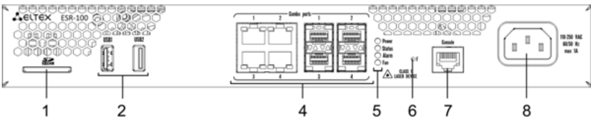
Рисунок 24 – Передняя панель ESR-100
