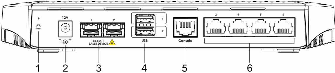
Рисунок 41 – Задняя панель ESR-15
