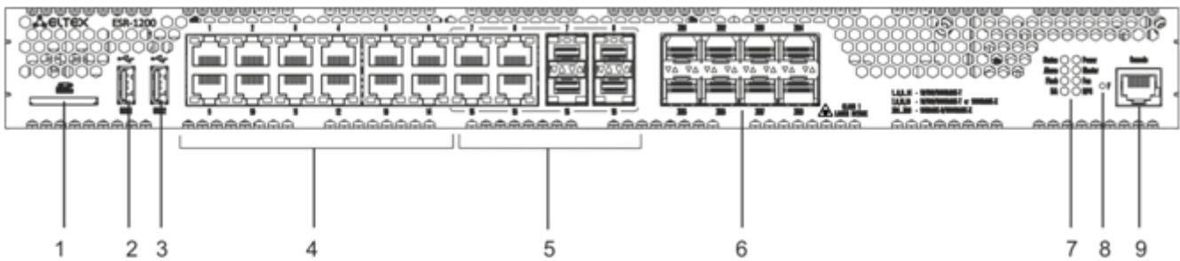
Рисунок 18 – Передняя панель ESR-1200
