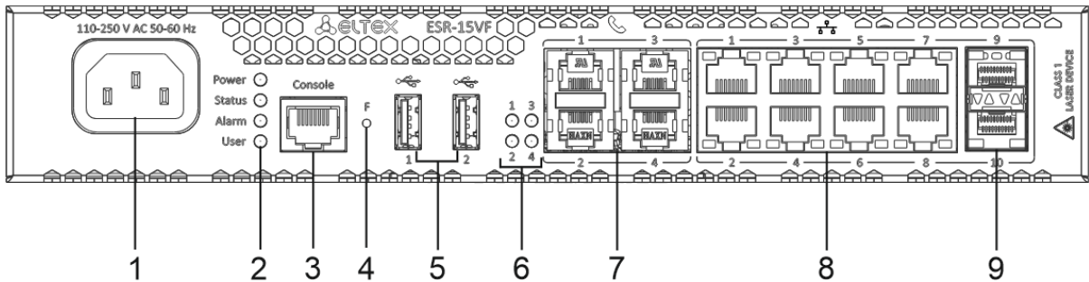
Рисунок 47 – Передняя панель ESR-15VF
