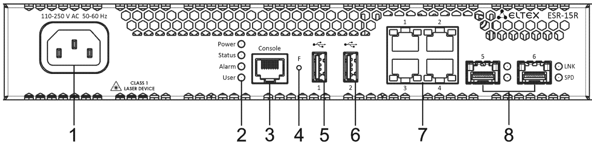
Рисунок 43 – Передняя панель ESR-15R
