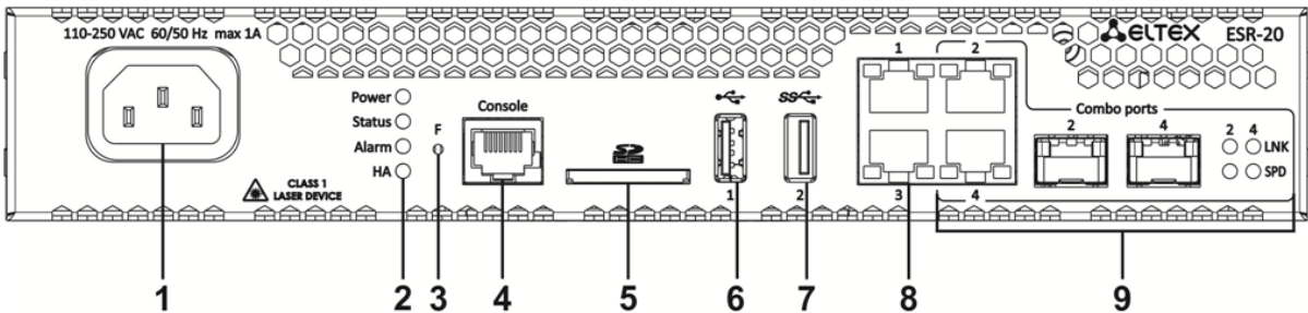
Рисунок 37 – Передняя панель ESR-20
