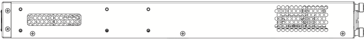
Рисунок 17 – Левая боковая панель ESR-1511, ESR-1500
