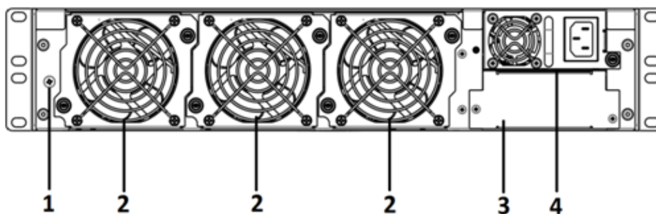
Рисунок 10 – Задняя панель ESR-1700
