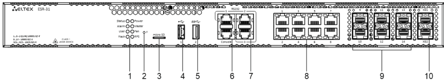
Рисунок 28 – Передняя панель ESR-31
