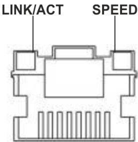
Рисунок 70 – Расположение индикаторов разъема RJ-45
