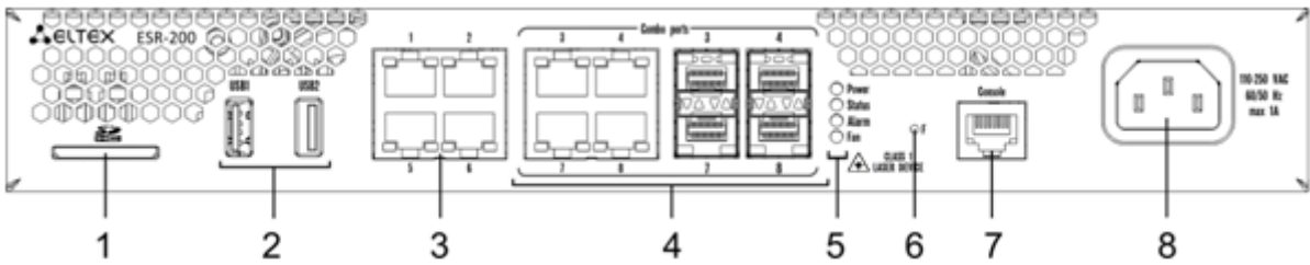
Рисунок 23 – Передняя панель ESR-200
