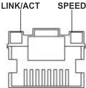
Рисунок 72 – Расположение индикаторов разъема RJ-45
