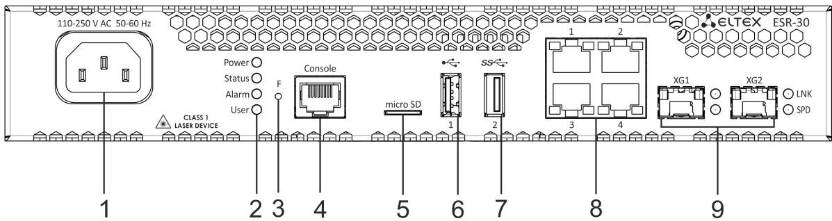
Рисунок 36 – Передняя панель ESR-30
