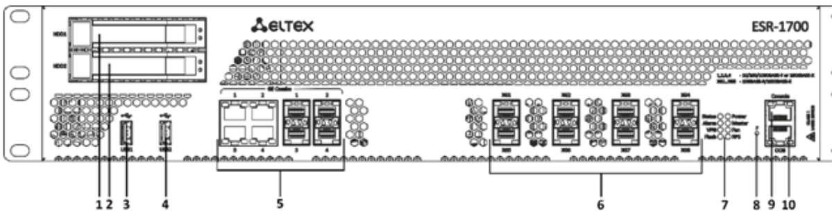
Рисунок 9 – Передняя панель ESR-1700
