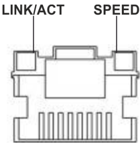
Рисунок 62 – Расположение индикаторов разъема RJ-45
