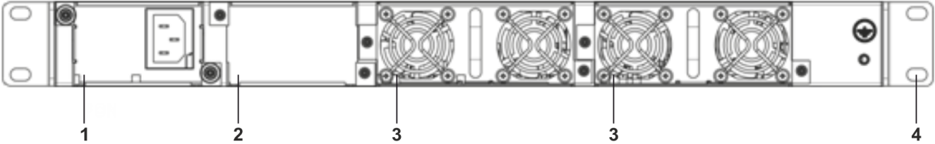
Рисунок 20 – Задняя панель ESR-1000
