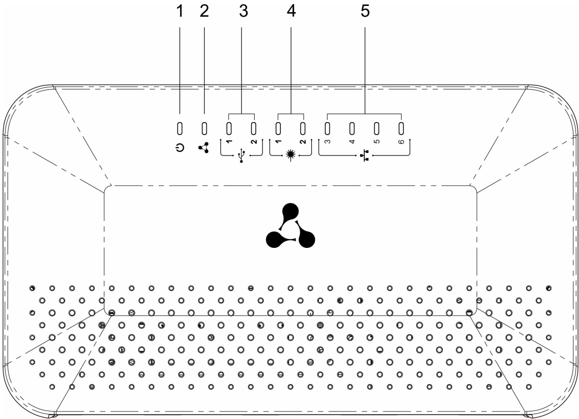
Рисунок 42 – Верхняя панель ESR-15
