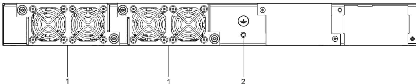
Рисунок 29 – Задняя панель ESR-31
