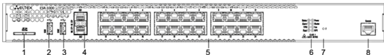
Рисунок 19 – Передняя панель ESR-1000
