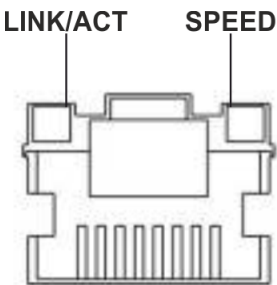
Рисунок 68 – Расположение индикаторов разъема RJ-45
