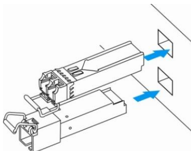
Рисунок 52 – Установка SFP-трансиверов
