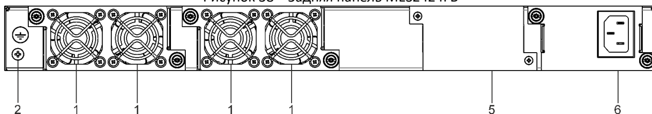
Рисунок 39 — Задняя панель MES3400-24, MES3400-48
