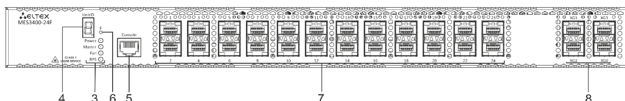
Рисунок 28 – Передняя панель MES3400-24F
