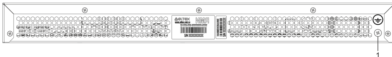
Рисунок 30 – Задняя панель MES1428, MES2428, MES2428T, MES2428B, MES2408IP DC1, MES2408P, MES2424 и MES2424B
