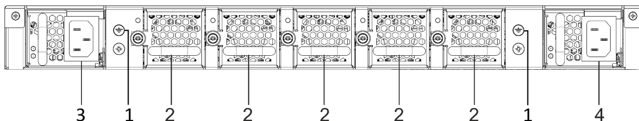
Рисунок 24 – Задняя панель MES5500-32
