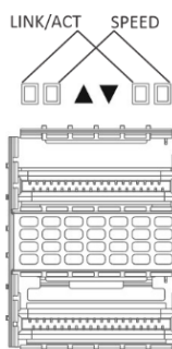
Рисунок 43 – Внешний вид разъема QSFP+ и QSFP28 для MES5400-xx
