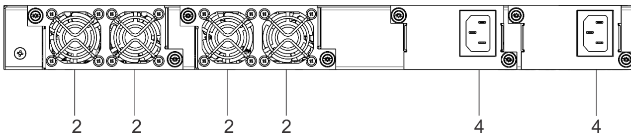
Рисунок 17 – Задняя панель MES3300-24
