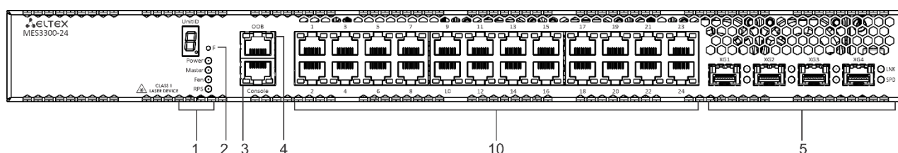
Рисунок 4 – Передняя панель MES3300-24
