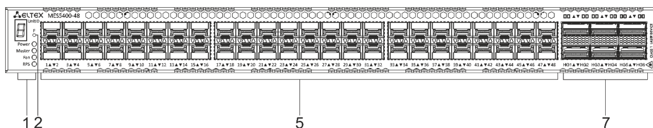
Рисунок 12 – Передняя панель MES5400-48
