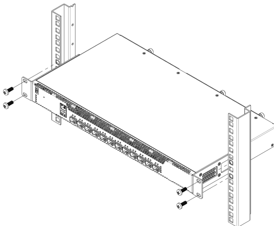
Рисунок 48 – Установка устройства в стойку
