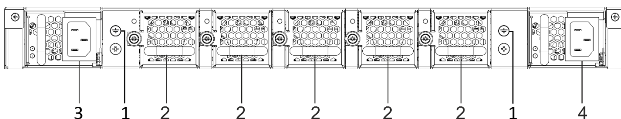
Рисунок 24 – Задняя панель MES5500-32
