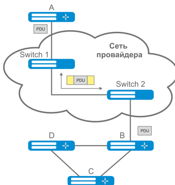
Рисунок 57 — Пример работы функции L2PT
