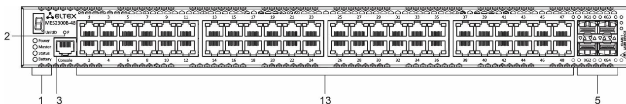
Рисунок 3 – Передняя панель MES2300B-48
