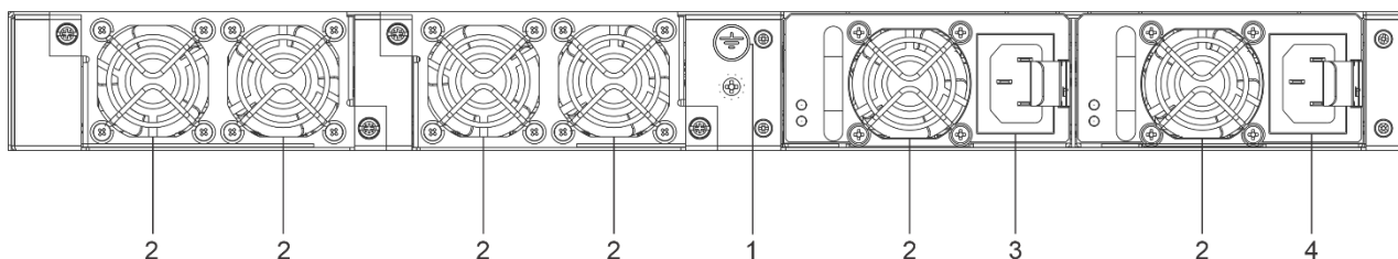
Рисунок 15 – Задняя панель MES2300-48P
