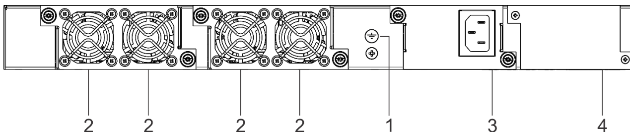
Рисунок 18 – Задняя панель MES3300-24F
