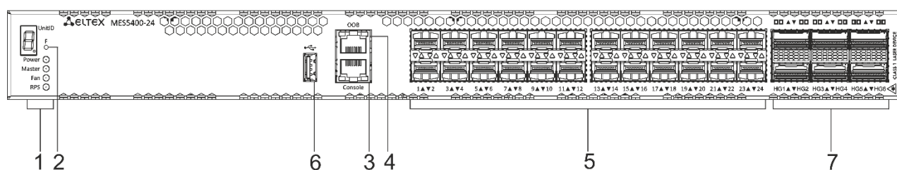
Рисунок 11 – Передняя панель MES5400-24
