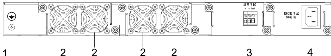
Рисунок 20 – Задняя панель MES5312, MES5324A, MES5332A
