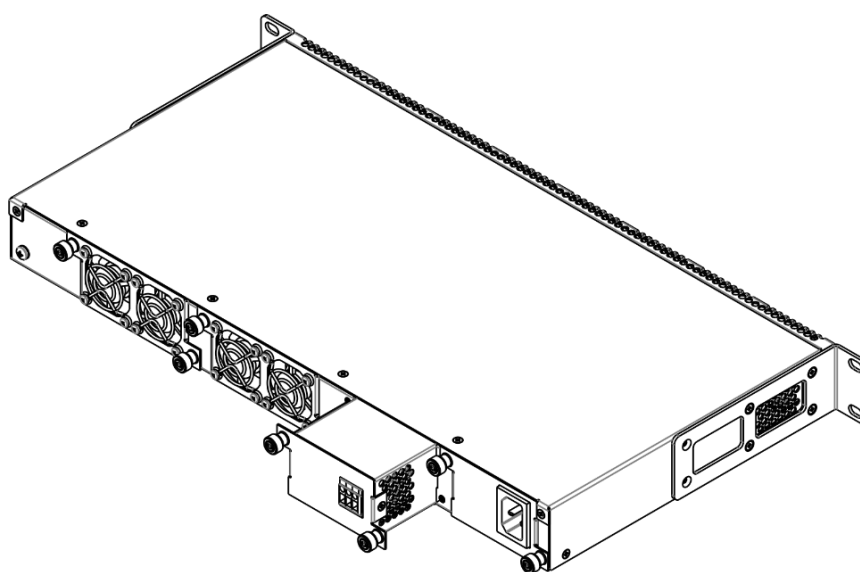
Рисунок 51 – Установка модулей питания
