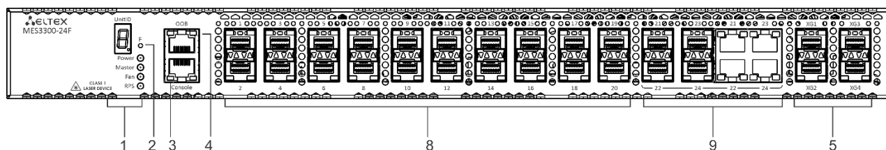
Рисунок 5 – Передняя панель MES3300-24F
