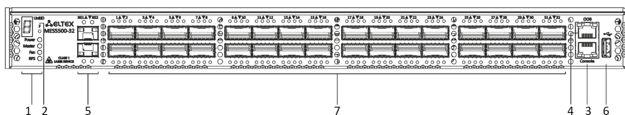
Рисунок 13 – Передняя панель MES5500-32
