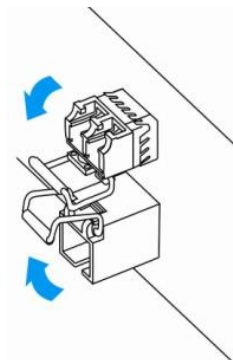
Рисунок 54 – Открытие защелки SFP-трансиверов
