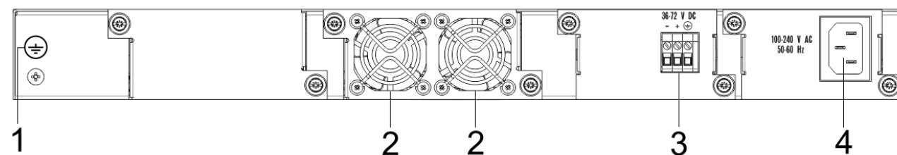
Рисунок 21 – Задняя панель MES5316A
