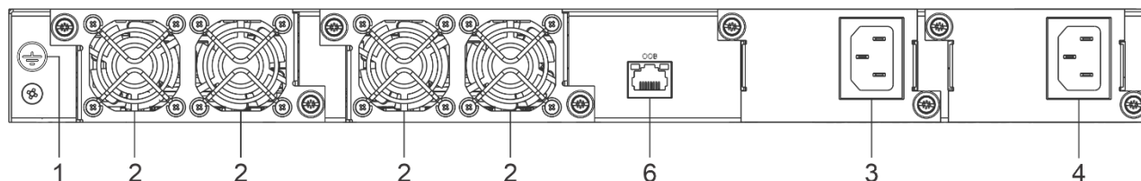
Рисунок 19 – Задняя панель MES3300-48
