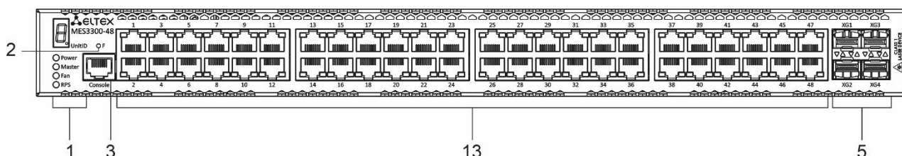
Рисунок 6 – Передняя панель MES3300-48
