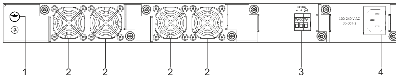
Рисунок 22 – Задняя панель MES5400-24
