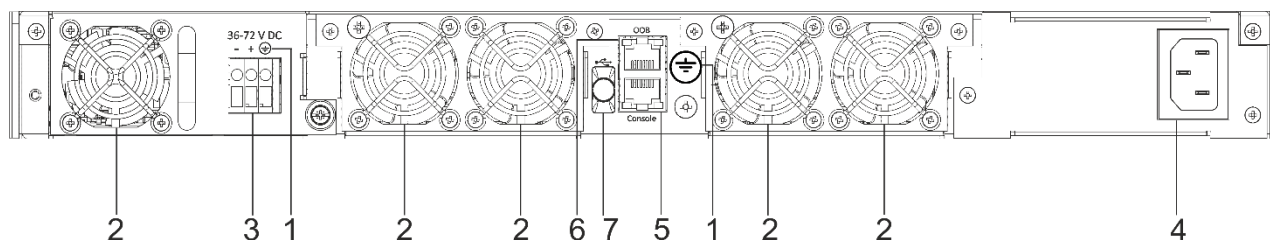
Рисунок 23 – Задняя панель MES5400-48
