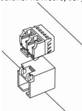
Рисунок 53 – Установленные SFP-трансиверы
