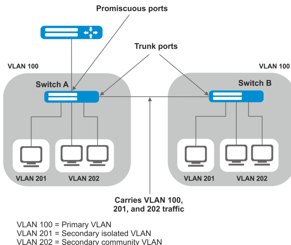
Рисунок 56 – Пример работы технологии Private VLAN
