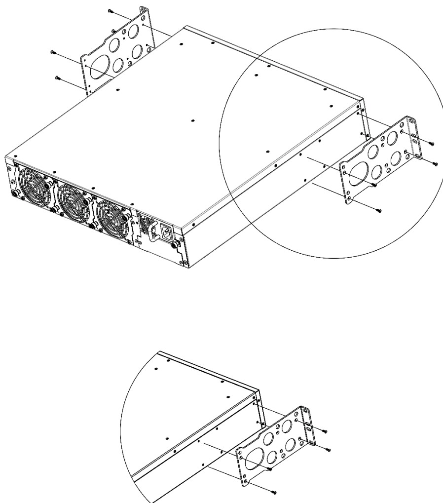
Рисунок 18 — Крепление кронштейнов
