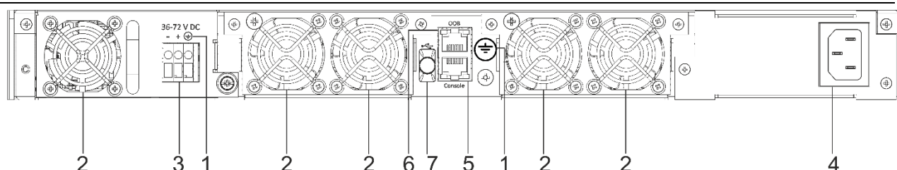
Рисунок 10 – Задняя панель MES5400-48
