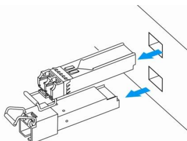
Рисунок 29 – Извлечение SFP-трансиверов
