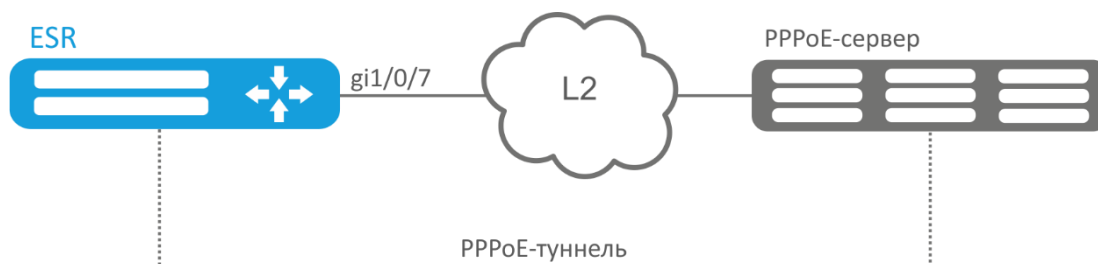
Рисунок 59 – Схема сети
