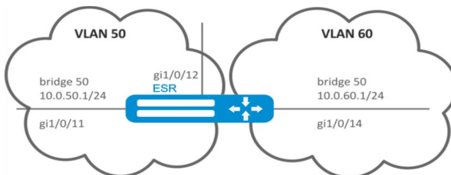
Рисунок 43 – Схема сети
