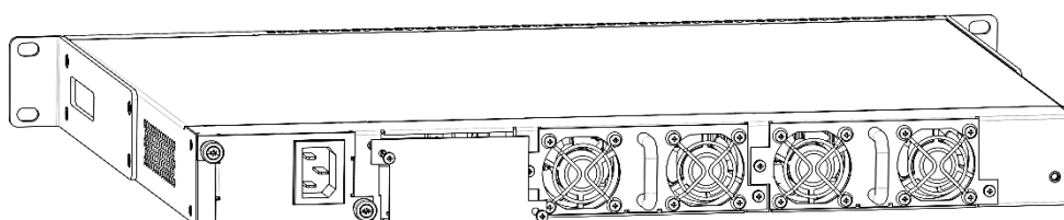
Рисунок 20 – Установка заглушки
