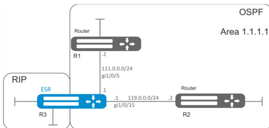
Рисунок 45 – Схема сети
