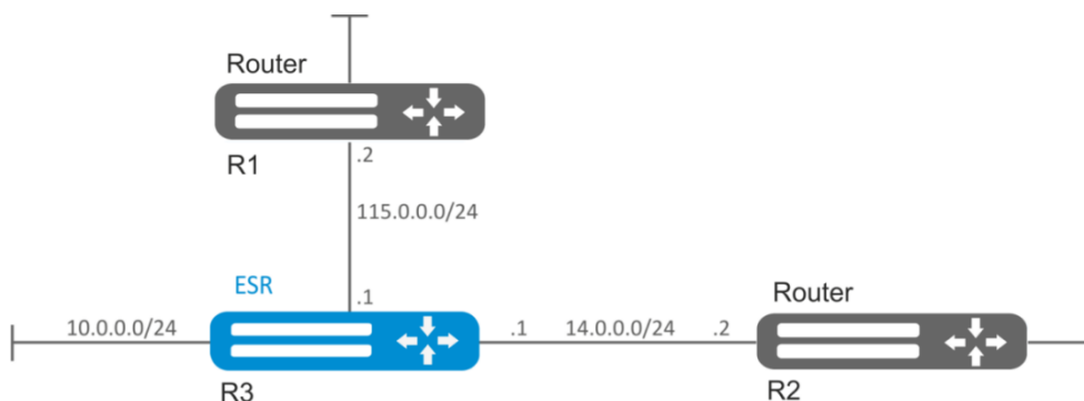
Рисунок 44 – Схема сети
