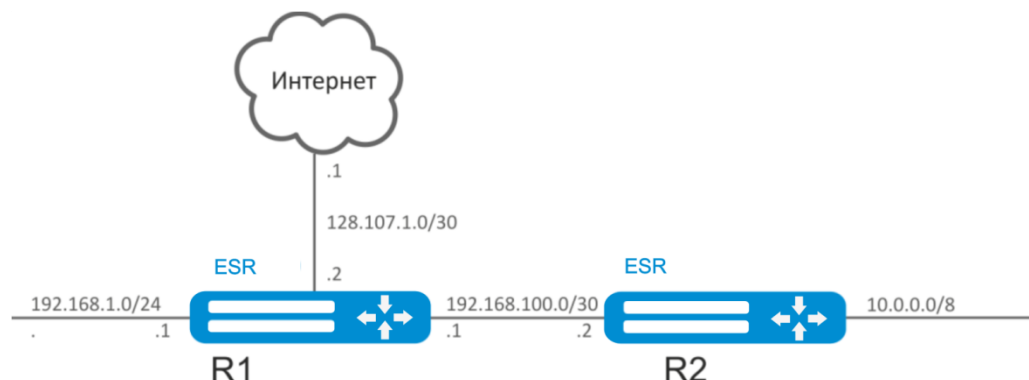
Рисунок 38 – Схема сети
