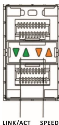
Рисунок 40 — Внешний вид разъема SFP/SFP+
