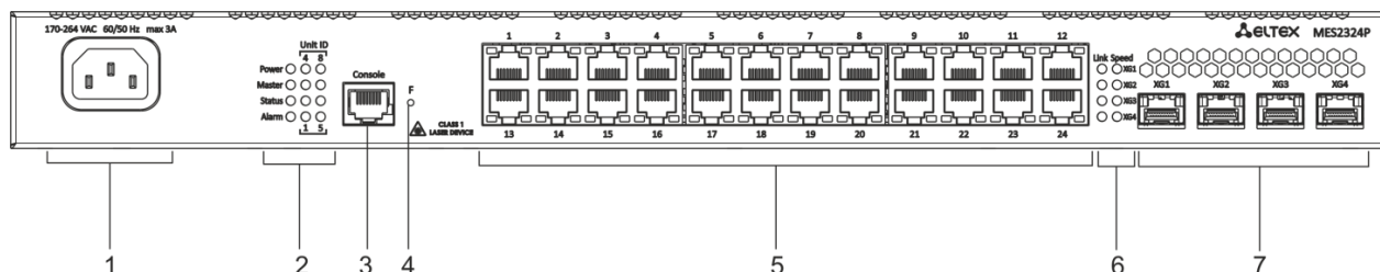
Рисунок 7 — Передняя панель MES2324P, MES2324P ACW
