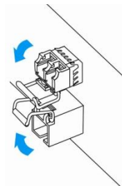
Рисунок 49 — Открытие защелки SFP-трансиверов
