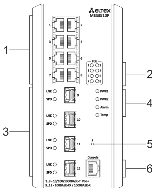
Рисунок 22 — Передняя панель MES3510P
