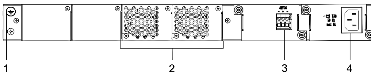
Рисунок 25 — Задняя панель MES3348
