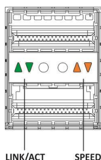
Рисунок 39 — Внешний вид разъема с QSFP+-трансиверами
