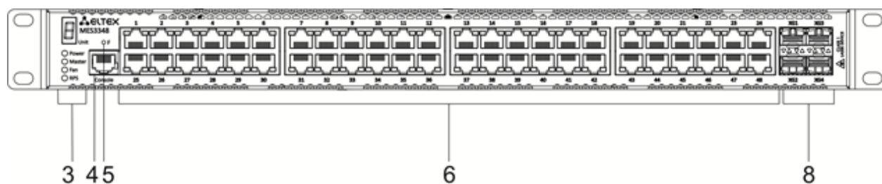
Рисунок 14 — MES3348, передняя панель
