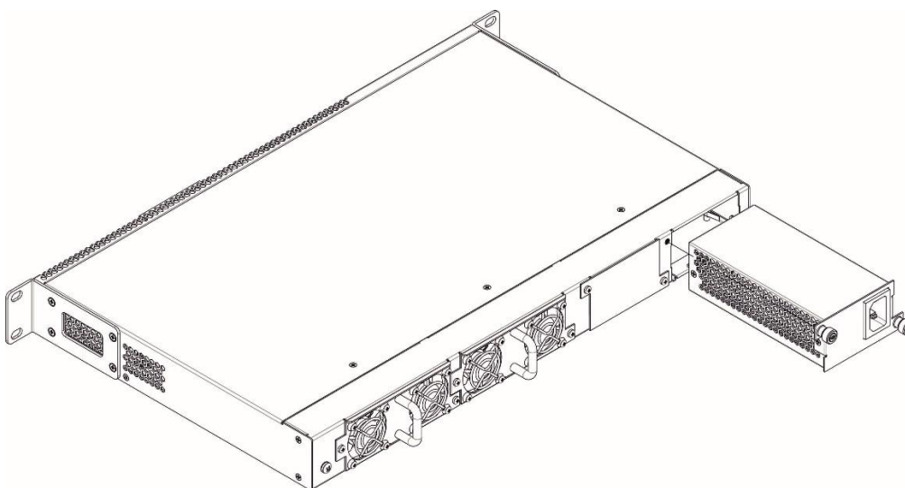
Рисунок 45 — Установка модулей питания
