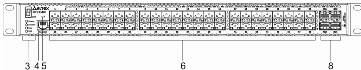
Рисунок 15 — MES3348F, передняя панель
