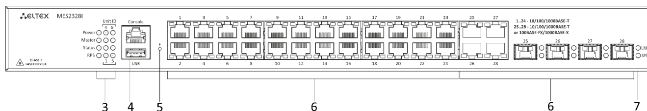
Рисунок 13 — MES2328I, передняя панель
