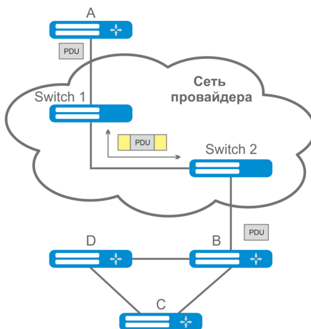
Рисунок 52 — Пример работы функции L2PT
