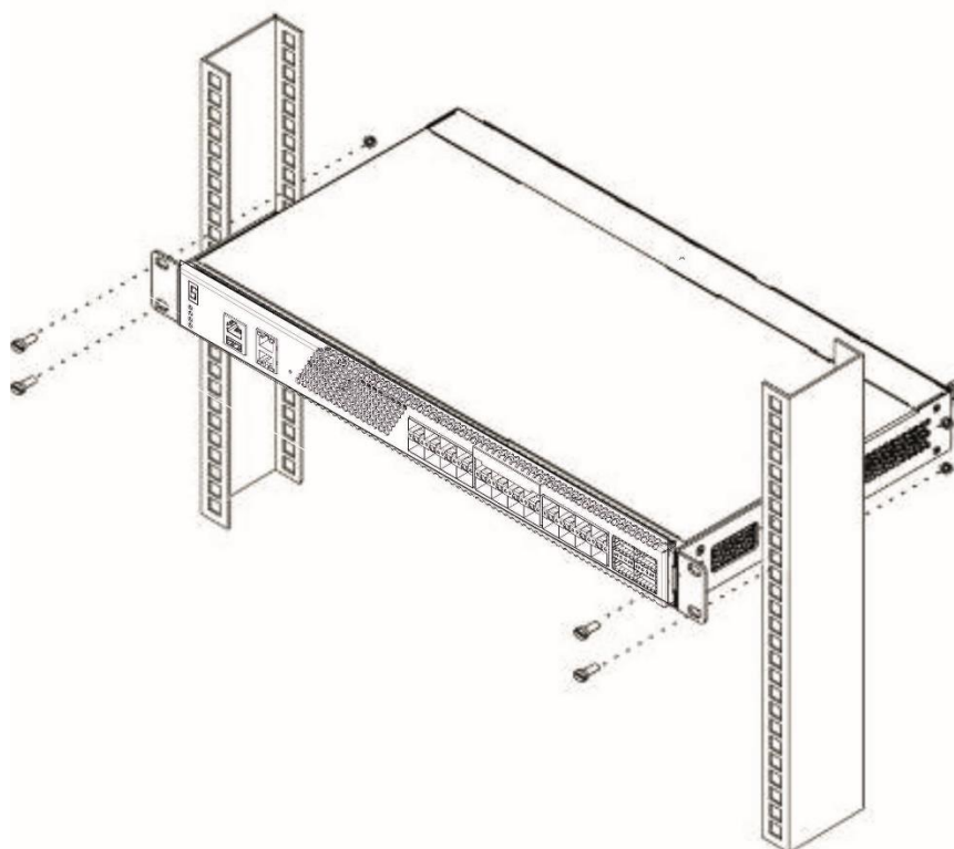
Рисунок 43 — Установка устройства в стойку
