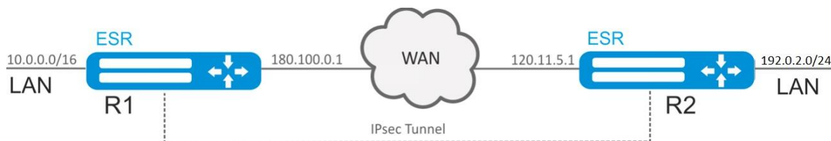
Рисунок 50 – Схема сети
