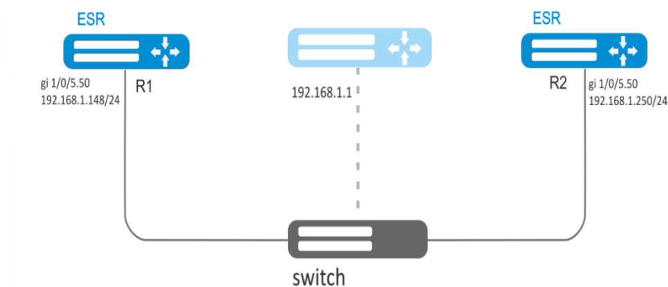
Рисунок 65 – Схема сети
