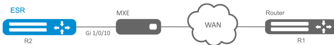
Рисунок 37 – Схема сети
