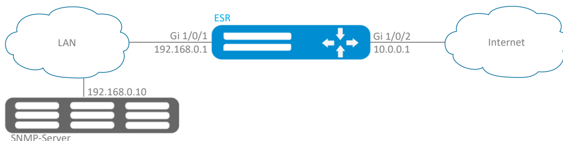
Рисунок 32 – Схема сети
