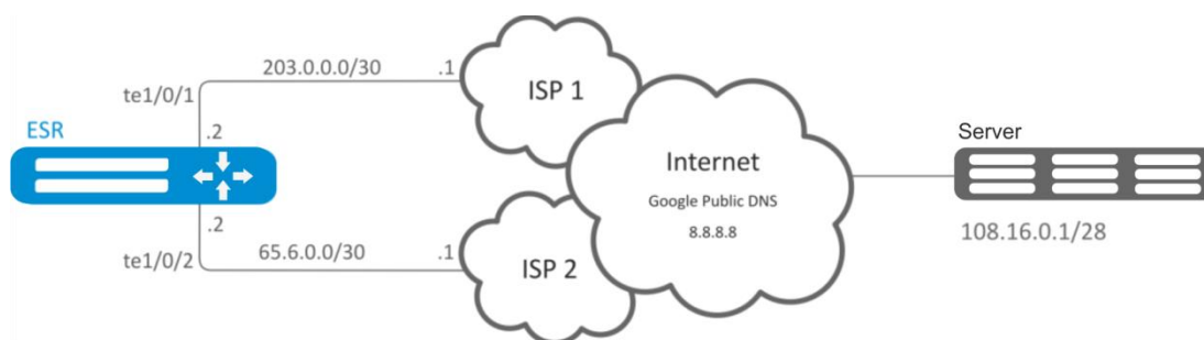
Рисунок 69 – Схема сети
