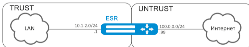
Рисунок 27 – Схема сети
