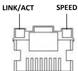
Рисунок 10 – Расположение индикаторов разъема RJ-45
