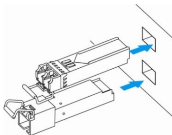
Рисунок 17 – Установка SFP-трансиверов
