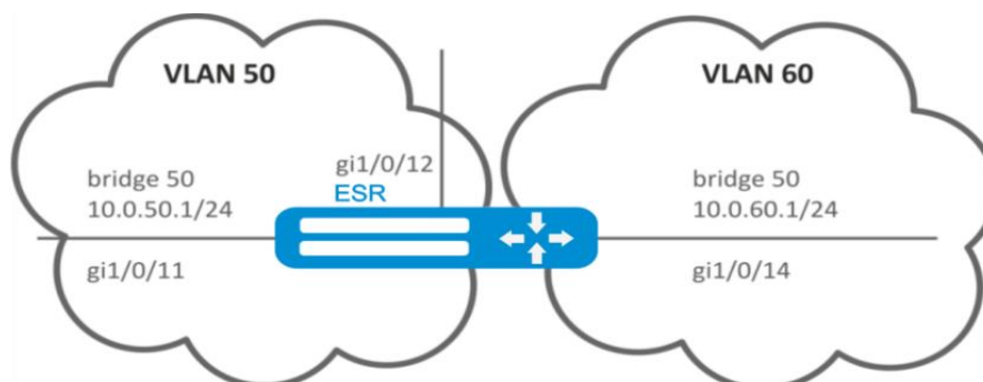
Рисунок 39 – Схема сети
