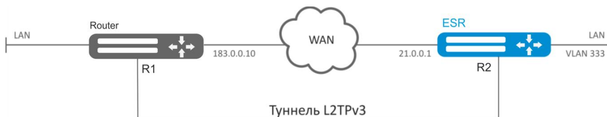
Рисунок 49 – Схема сети
