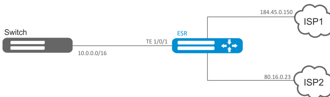
Рисунок 47 – Схема сети
