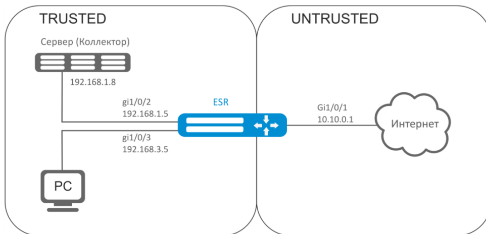
Рисунок 63 – Схема сети
