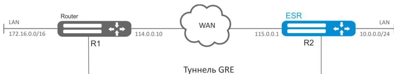
Рисунок 48 – Схема сети
