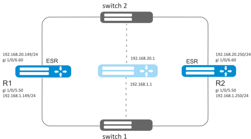
Рисунок 66 – Схема сети
