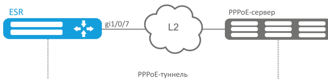
Рисунок 55 – Схема сети
