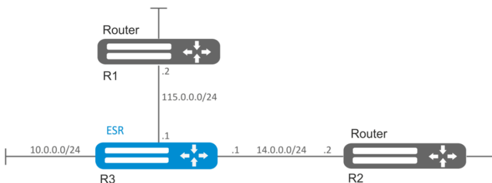
Рисунок 40 – Схема сети
