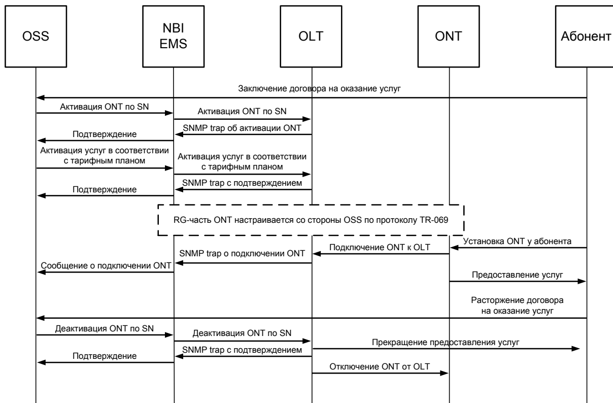
Рисунок 2а – Схема обмена сообщениями между OSS и ONT при активации ONT до установки абоненту
