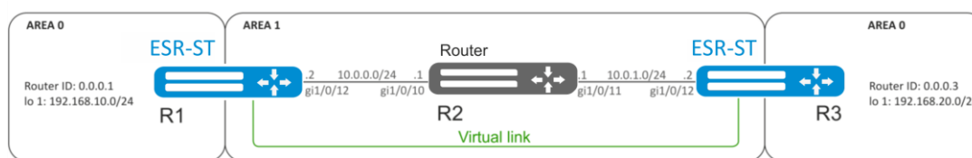
Рисунок 9.15 – Схема сети
