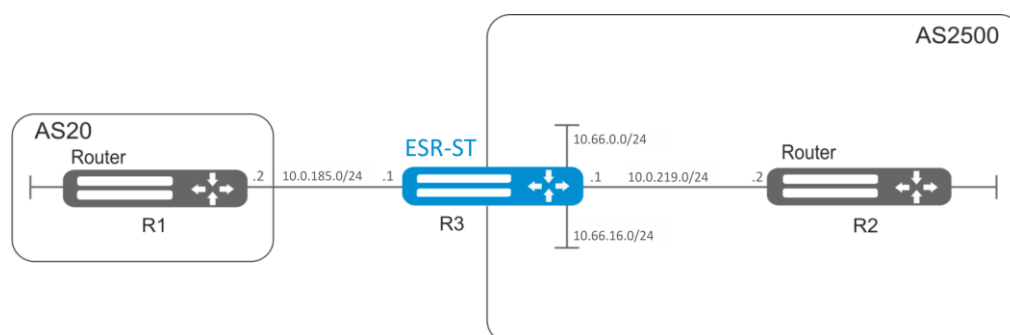
Рисунок 9.16 – Схема сети
