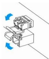
Рисунок 6.7 – Открытие защелки SFP-трансиверов
